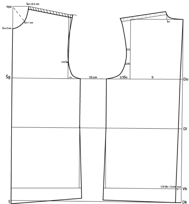
Slika 13. Konstrukcija prednjeg i stražnjeg dijela ženske bluze
