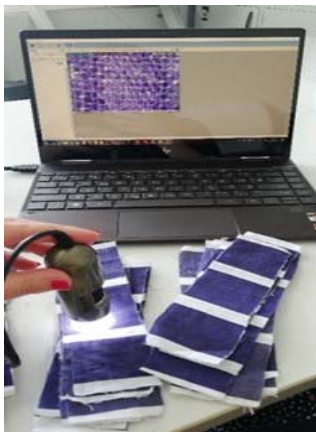
Slika 46. Mjerenje uzoraka pomoću Dino-Lite digitalnog mikroskopa
