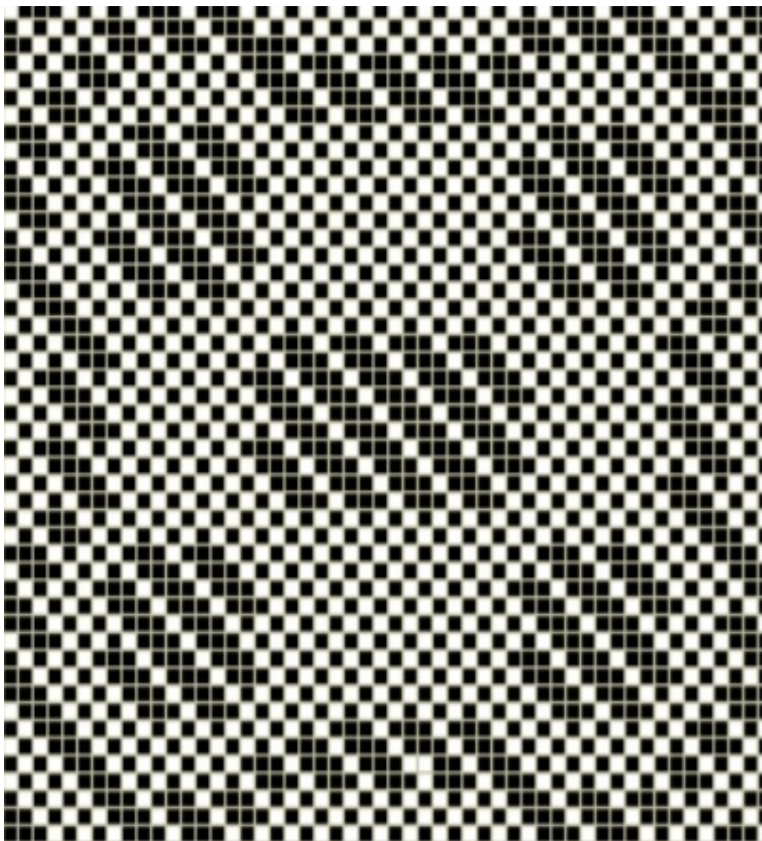
Sl. 15. Jedinica veza tkanine
