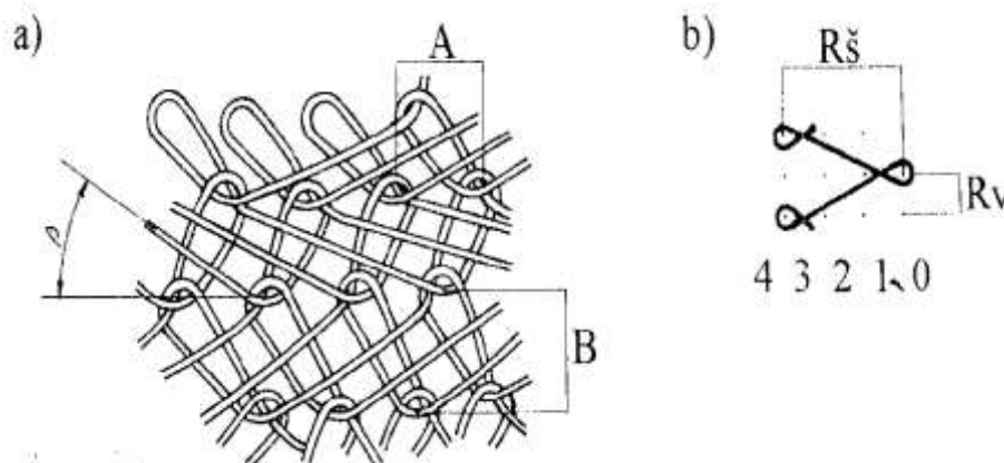
Sl. 10 Pousaten vez: a) preplet (A- korak očice, B- visina očice), b) slijed niti, R_s – širinski raport, R_v – visinski raport
