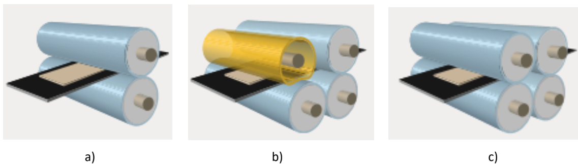
Sl.5 Tlačni sustavi u strojevima tt. Kannegieser i Veit: a) Standardni tlačni sustav; b) Flexo tlačni sustav; c) Dvojni tlačni sustav [8]
