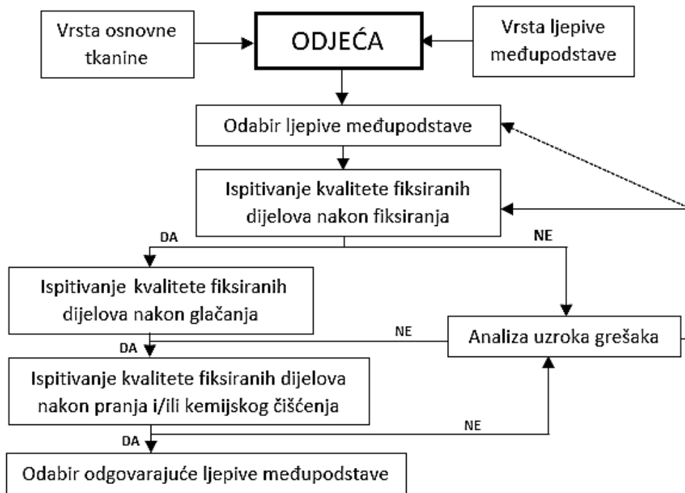
Sl.6 Dijagram toka za odabir ljevne međupodstave [9]
