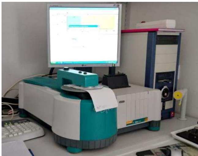
Slika 14. Transmisijски спектрофотометар Cary 50/Soloscreen (Varian)
