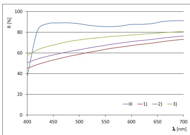
SI.12. Remisijske krivulje kemijski bijeljenog platna, tiskanog čistim pastama
