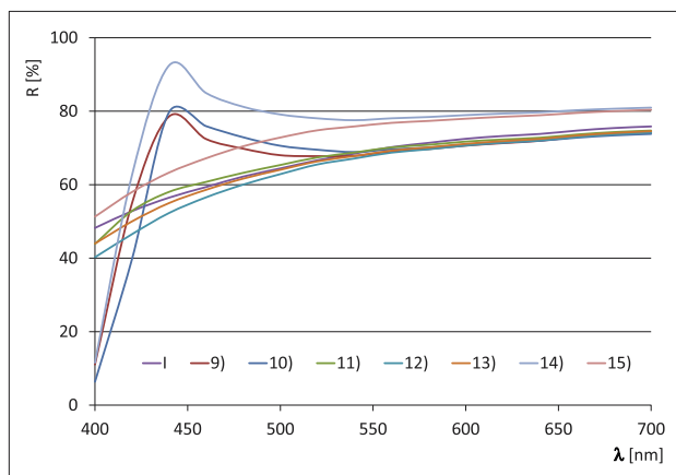
SI.8 Remisijske krivulje platna opranog tenzidom, tiskanog kombinacijom pasta uz dodatak fluorescentnog optičkog bjelila i fosforescentnog pigmenta
