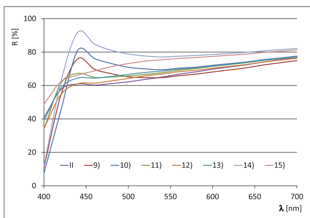
SI.11 Remisijske krivulje platna opranog komercijalnim deterdžentom, tiskanog kombinacijom pasta uz dodatak fluorescentnog optičkog bjelila i fosforescentnog pigmenta
