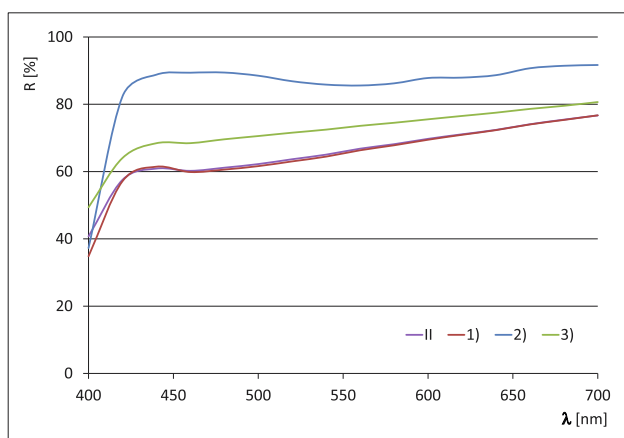
SI.9 Remisijske krivulje platna opranog komercijalnim deterdžentom, tiskanog čistim pastama
