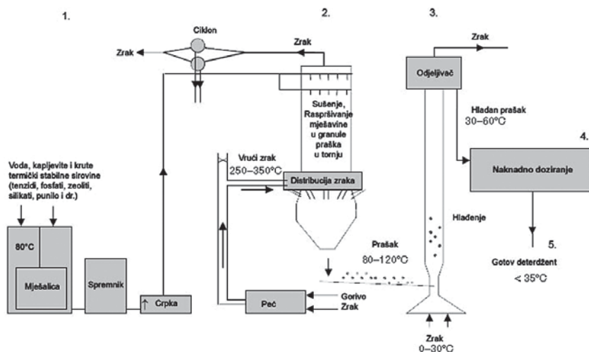
Sl.1 Shematski prikaz proizvodnje deterdženta postupkom raspršivanja vrućim zrakom: 1. Dobivanje smjese za raspršivanje; 2. Raspršivanje smjese u granule praška (osnovni prašćak ili raspršena smjesa); 3. Ujednaćavanje čestica osnovnog praška; 4. Naknadno doziranje sirovina; 5. Pakiranje [6]
