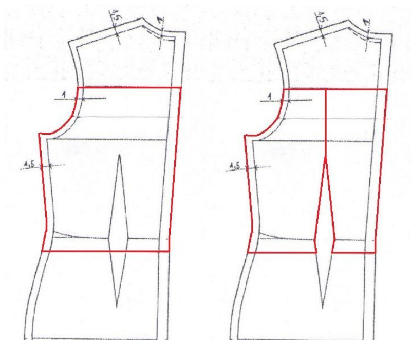
Slike 13. i 14. Modeliranje stražnjeg dijela kroja
