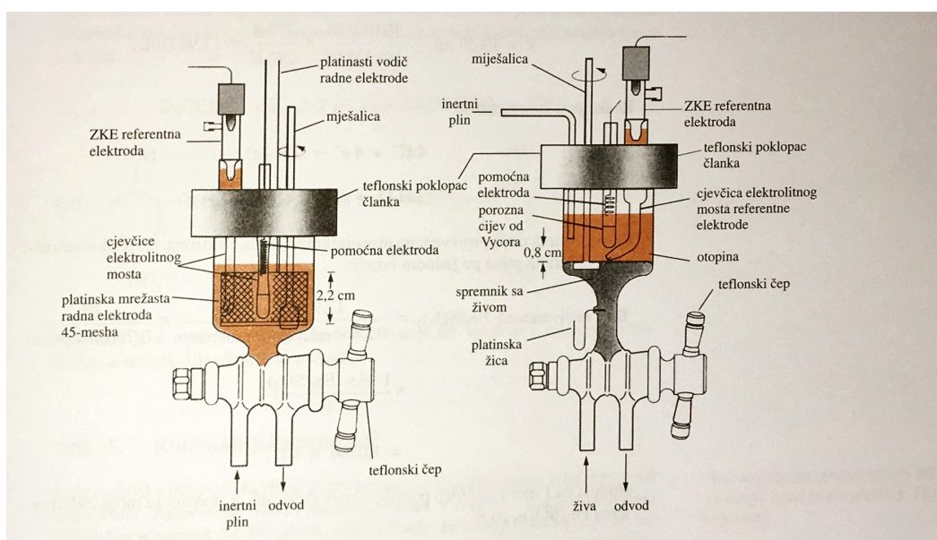
slika 4. Elektrolitički članak za potenciometrijsku kulometriju [4]
