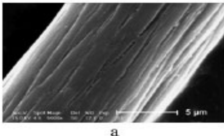
Slika 12. Prikaz PAN vlakna prije obrade titanovim dioksidom [20]
