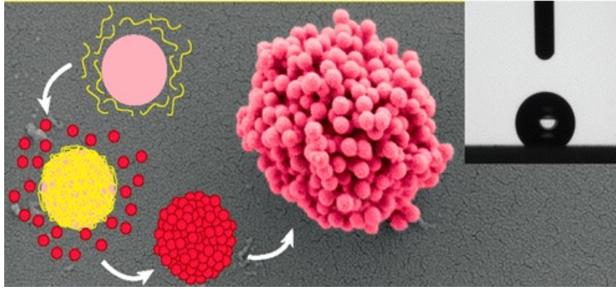
slika 10. Malina čestice [26]
