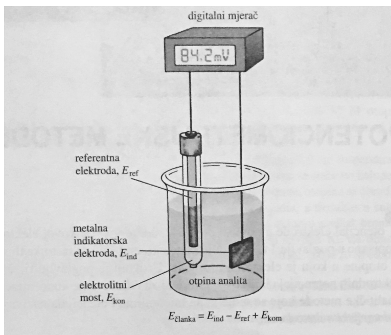
Slika 2. Članak za potenciometrijske analize [4]
