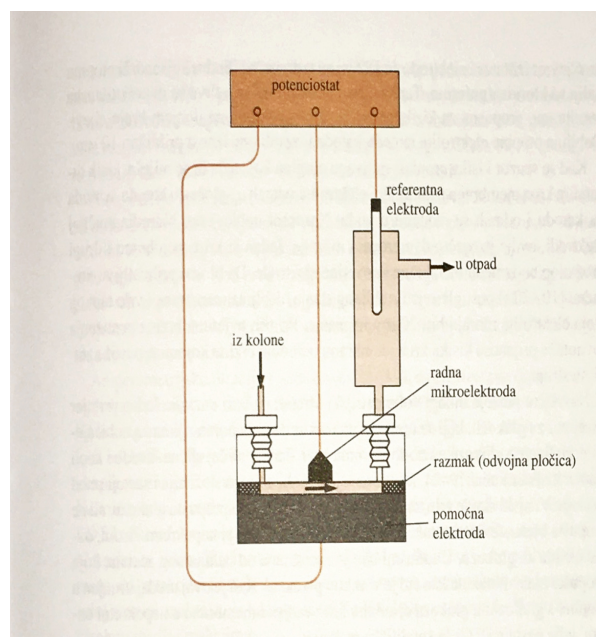
Slika 3. Voltametrijoski sustav za određivanje spojeva na izlasku iz kolone [4]
