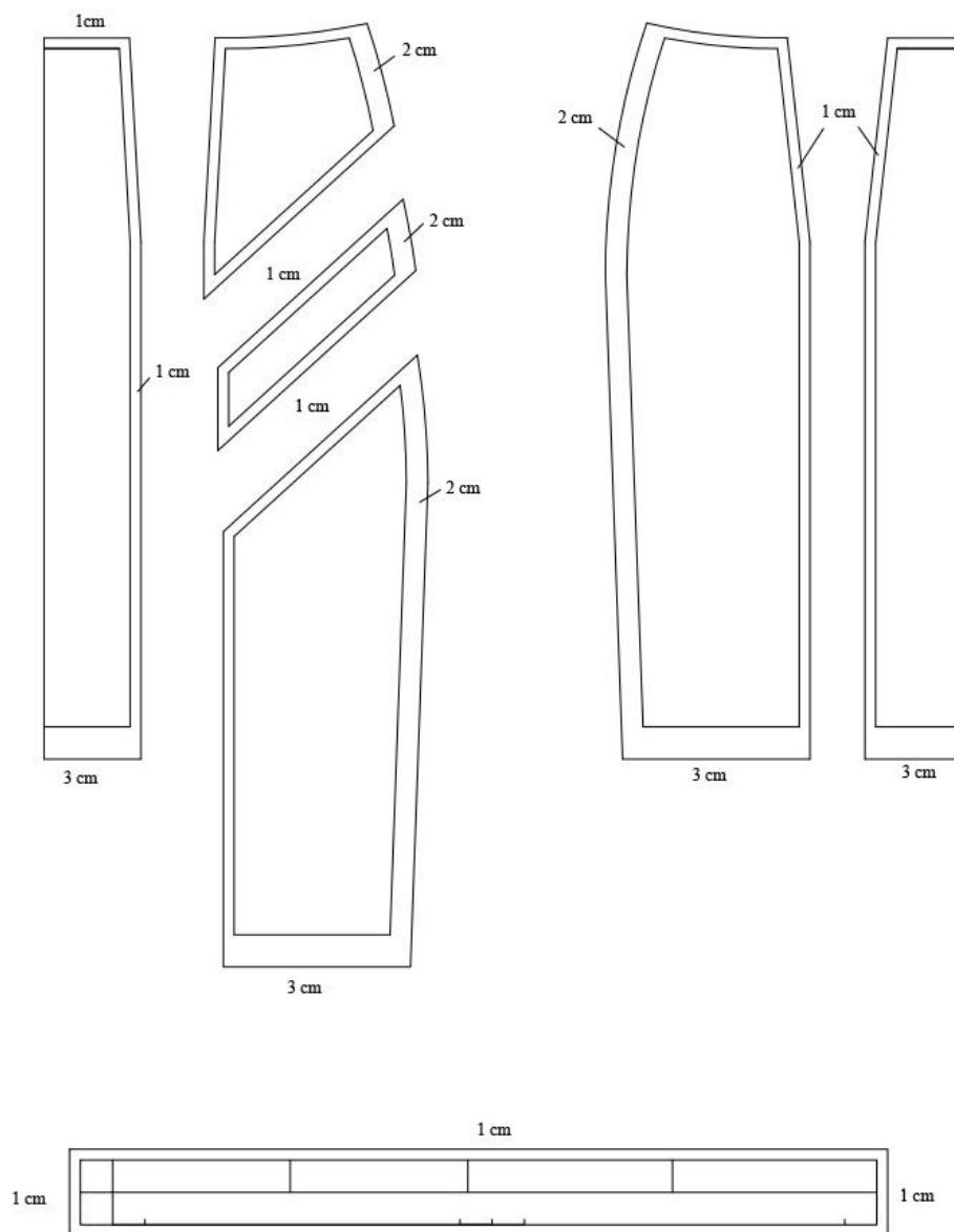
Slika 19: Dodavanje šavnih dodataka na krojne dijelove ženske suknje
