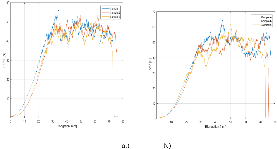
Slika 26. Ispis rezultata u obliku grafičkog prikaza sile, a) koža 2 (leđni dio), smjer centralne osi, b) koža 2 (leđni dio) okomito na smjer centralne osi
