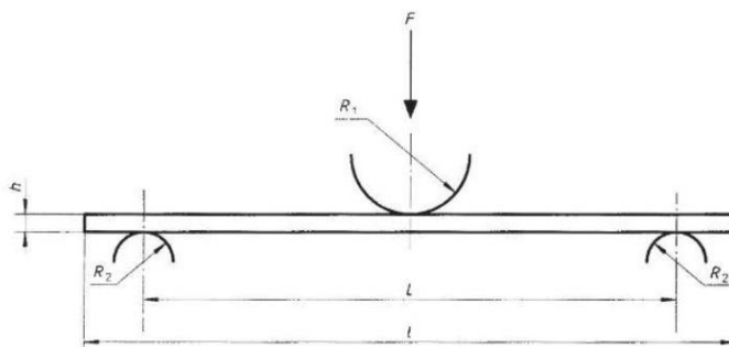
Slika 30. Skica ispitivanja savojne čvrstoće [34]
