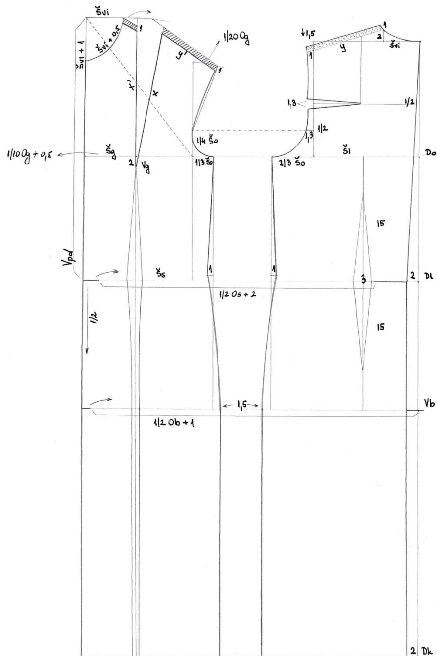
Sl. 15. Prikaz konstrukcije temeljnog kroja za haljinu
