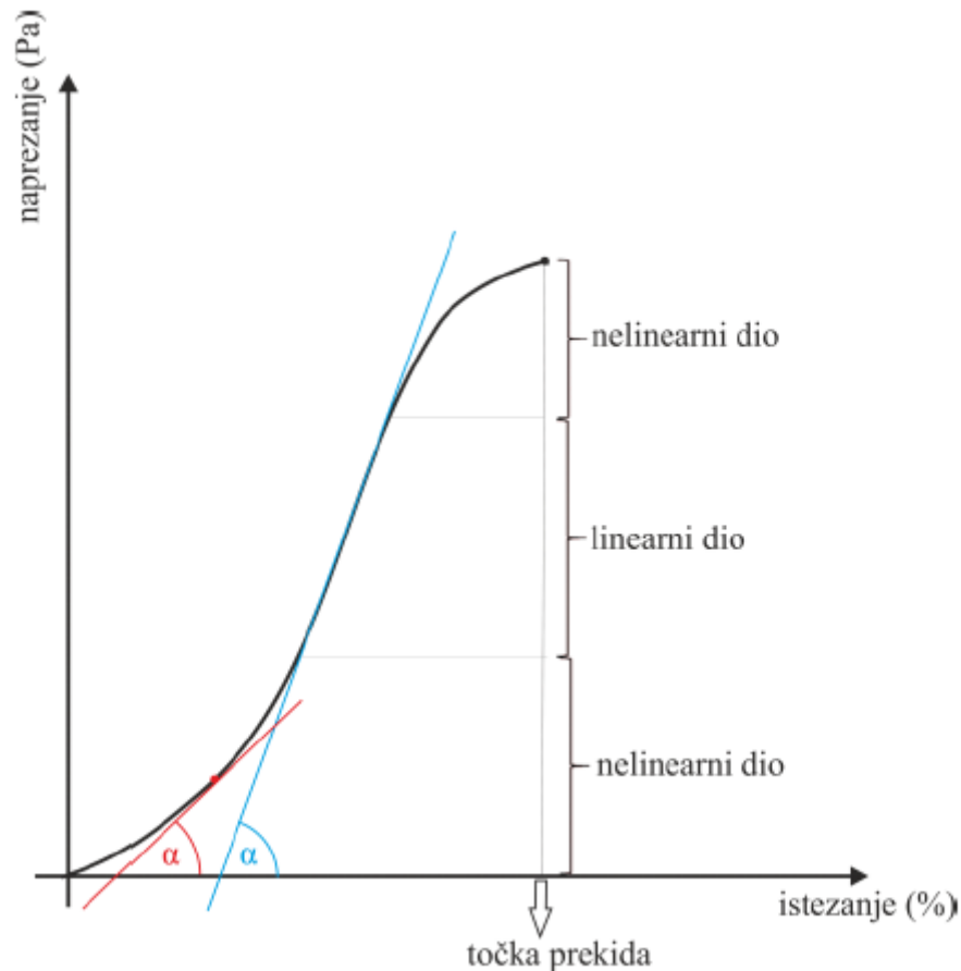
Sl. 9. Tipična krivulja naprezanje/istežanje za tkanine [ 4 ].
