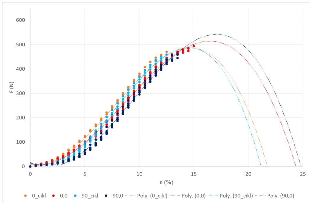
SI. 30. Vlačno ponašanje tkanine u poprečnom rips vezu (24/24) prije i nakon cikličkog naprezanja
