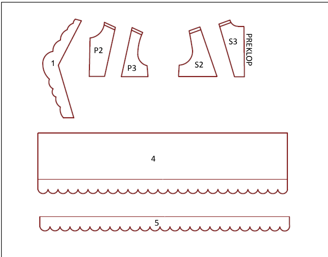
Slika 55. Krojni dijelovi
