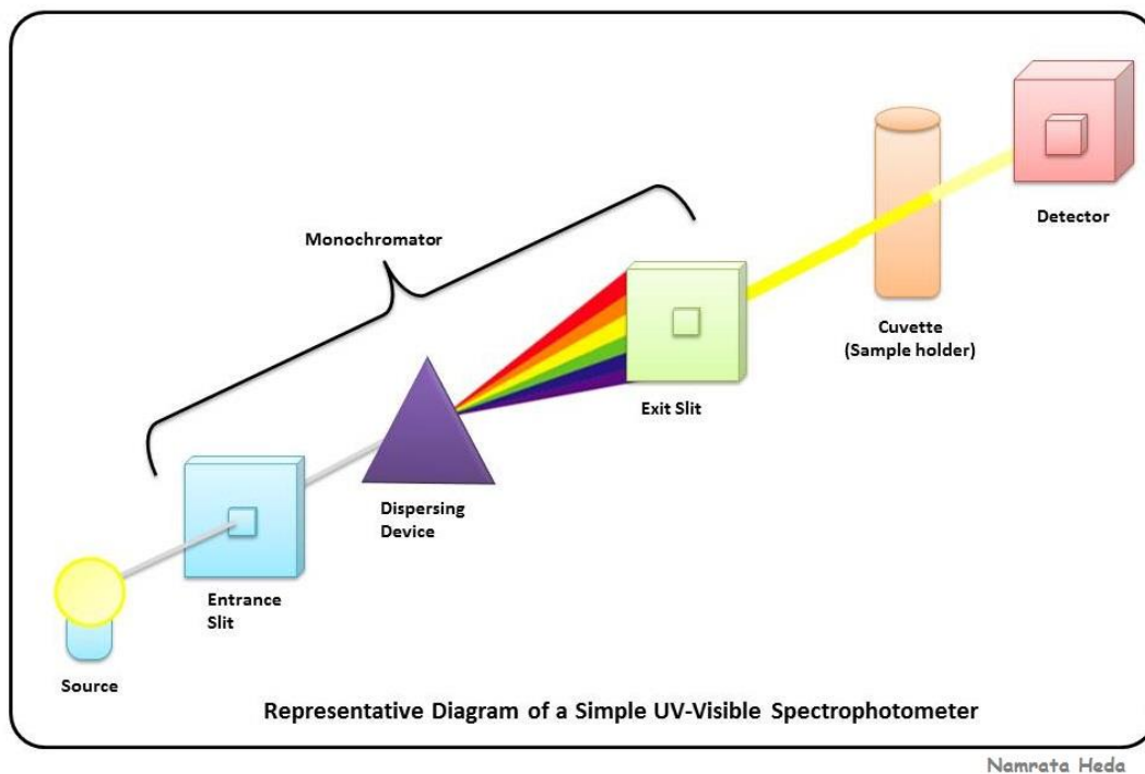
Slika 11. Dijagram jednostavnog UV-V vidljivog spektrofotometra
