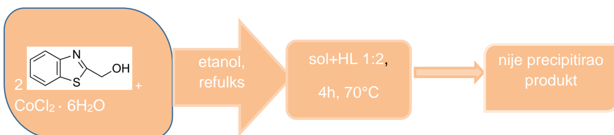
Schema 3. Prikaz sinteze \text{CoCl}_2 \cdot 6\text{H}_2\text{O} i HL u molarnom omjeru 1:2
