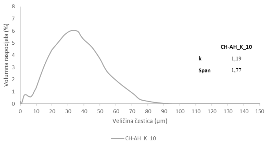
Slika 121. Raspodjela veličina čestica u efluentima za 10 ciklusa pranja poliester/kitozan strukture pripravljene konvencionalnim predobradama alkalnom hidrolizom uz dodatak promotora
