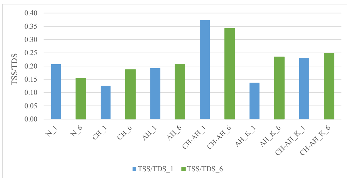
Slika 83. Omjer ukupne suspendirane i ukupne otopljene tvari u efluentima od pranja konvencionalnim predobradama dobivene poliestera/kitozana strukture tijekom 1 – 5 i 6 – 10 ciklusa pranja
