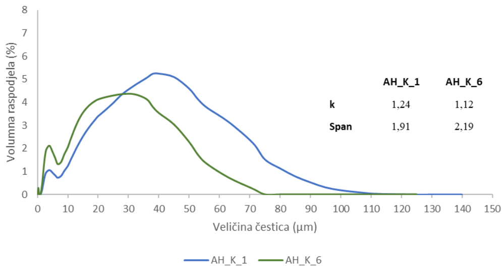
Slika 89. Raspodjela veličina čestica u efluentima od 1 – 5 i 6 – 10 ciklusa pranja alkalno hidrolizirane poliesterske tkanine uz dodatak promotora
