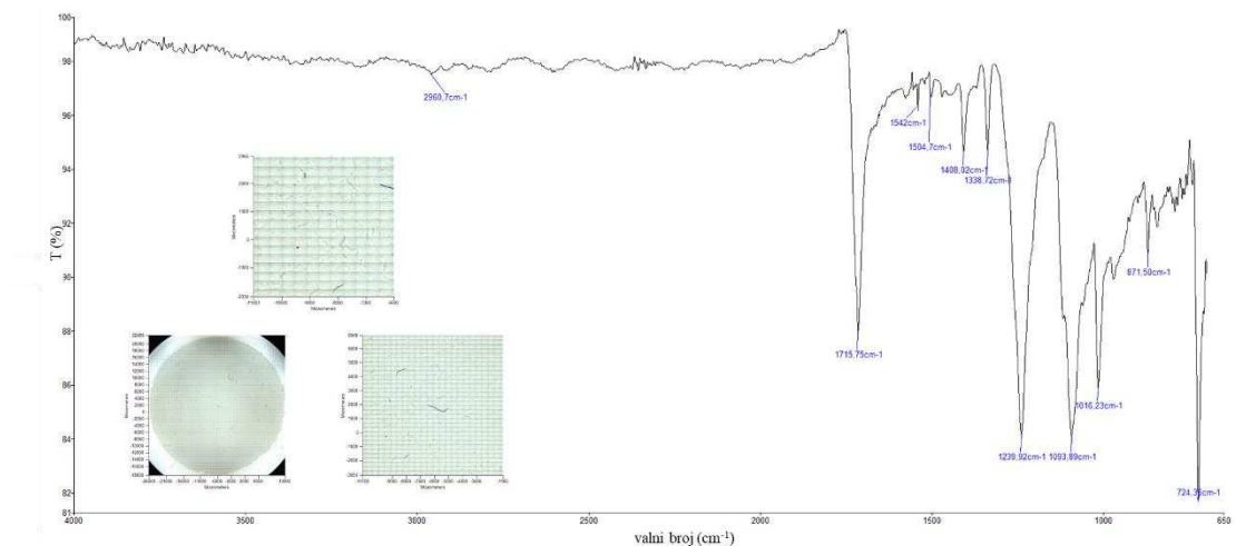
Slika 110. FTIR spekter i mikroskopske slike filtra nakon filtracije efluenta (10 ciklusa pranja) standardne polieterske tkanine predobrađene alkalnom hidrolizom uz dodatak kationskog tenzida
