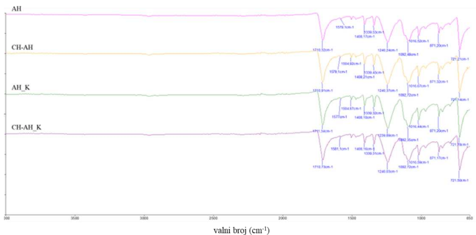
Slika 50. FTIR spektar alkalno predobrađenih i kitozanom modificiranih poliesterskih tkanina
