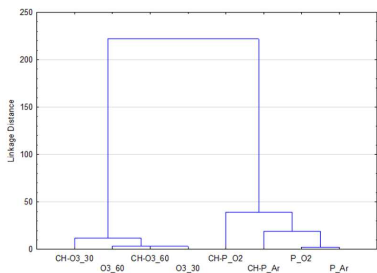
Slika 62. Dendrogram HCA provedene na osnovi fizikalno-mehaničkih svojstava za poliesterske tkanine predobrađene naprednim postupcima i modificirane kitozanom
