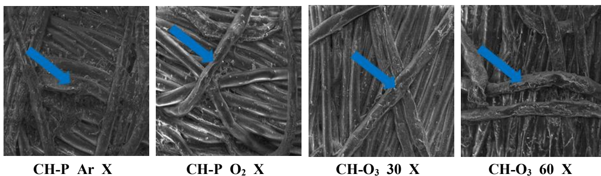
Slika 75. SEM slike nakon 10 ciklusa pranja napredno predobrađene poliesterne tkanine modificirane kitozonom
