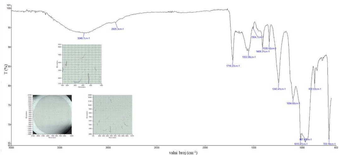
Slika 114. FTIR spekter i mikroskopske slike filtra nakon filtracije efluenta (10 ciklusa pranja) kitozonom modificirane standardne polieterske tkanine predobrađene ozonom u vremenu od 30 minuta
