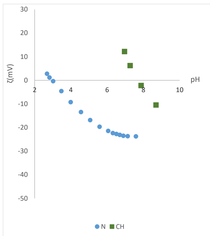
Slika 45. Krivulja zeta potencijala neobrađene i kitozanom modificirane poliesterske tkanine u ovisnosti o pH 1 mmol/L KCl
