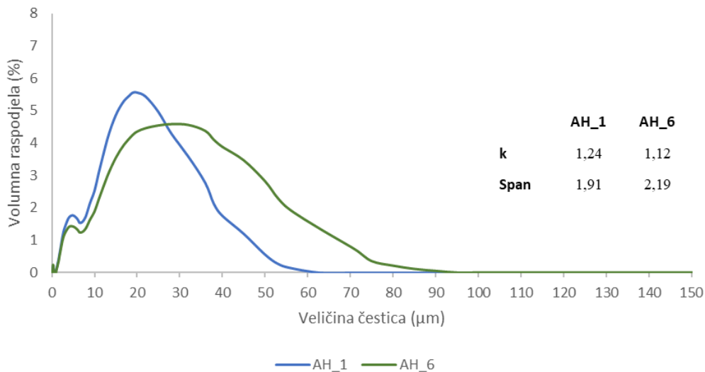
Slika 88. Raspodjela veličina čestica u efluentima za 1 – 5 i 6 – 10 ciklusa pranja alkalno hidrolizirane poliesterske tkanine
