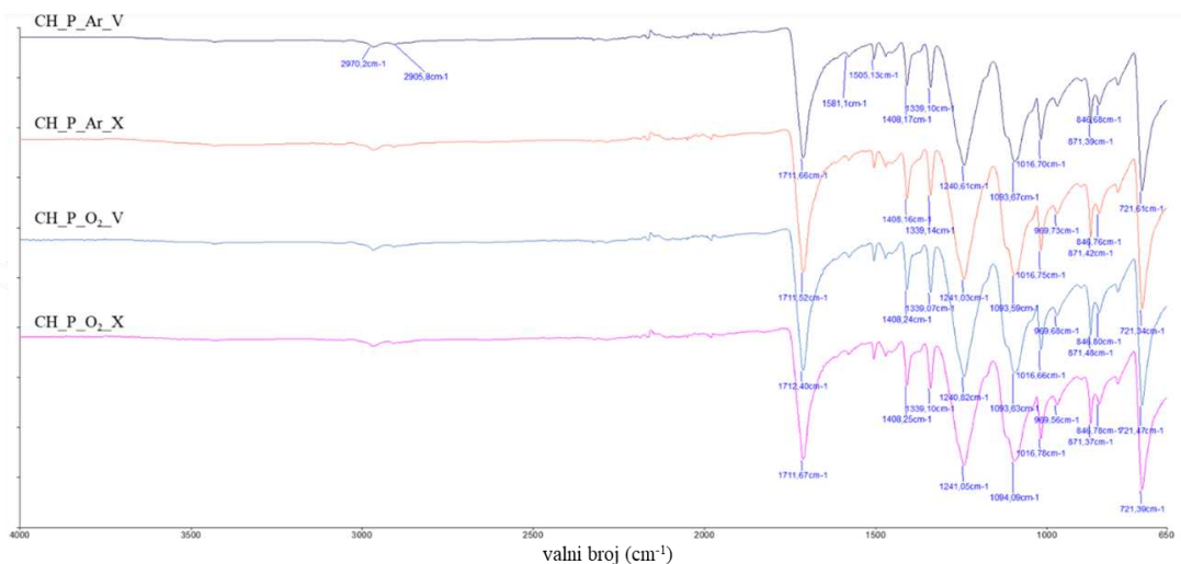
Slika 70. FTIR spektar plazmom predobrađene poliesterske tkanine modificirane kitozanom nakon 5 i 10 ciklusa pranja
