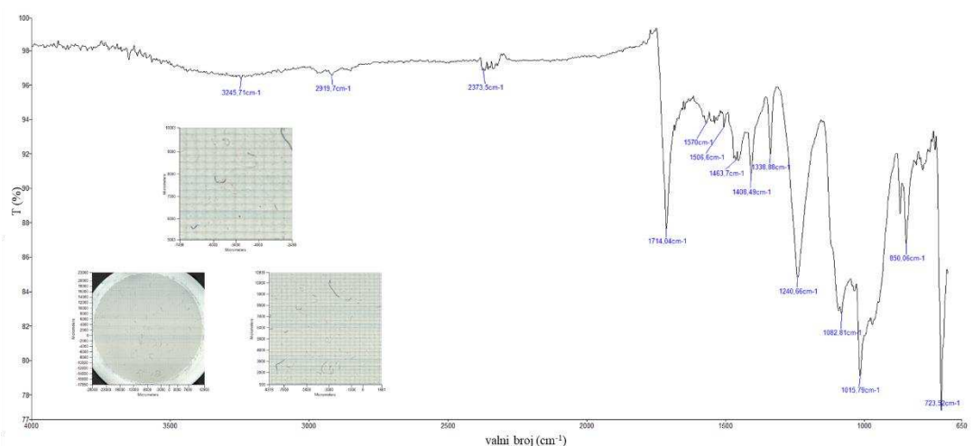
Slika 115. FTIR spekter i mikroskopske slike filtra nakon filtracije efluenta (10 ciklusa pranja) kitozonom modificirane standardne polieterske tkanine predobrađene ozonom u vremenu od 60 minuta
