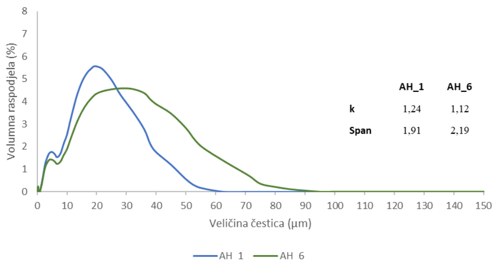
Slika 88. Raspodjela veličina čestica u efluentima za 1 – 5 i 6 – 10 ciklusa pranja alkalno hidrolizirane polieterske tkanine
