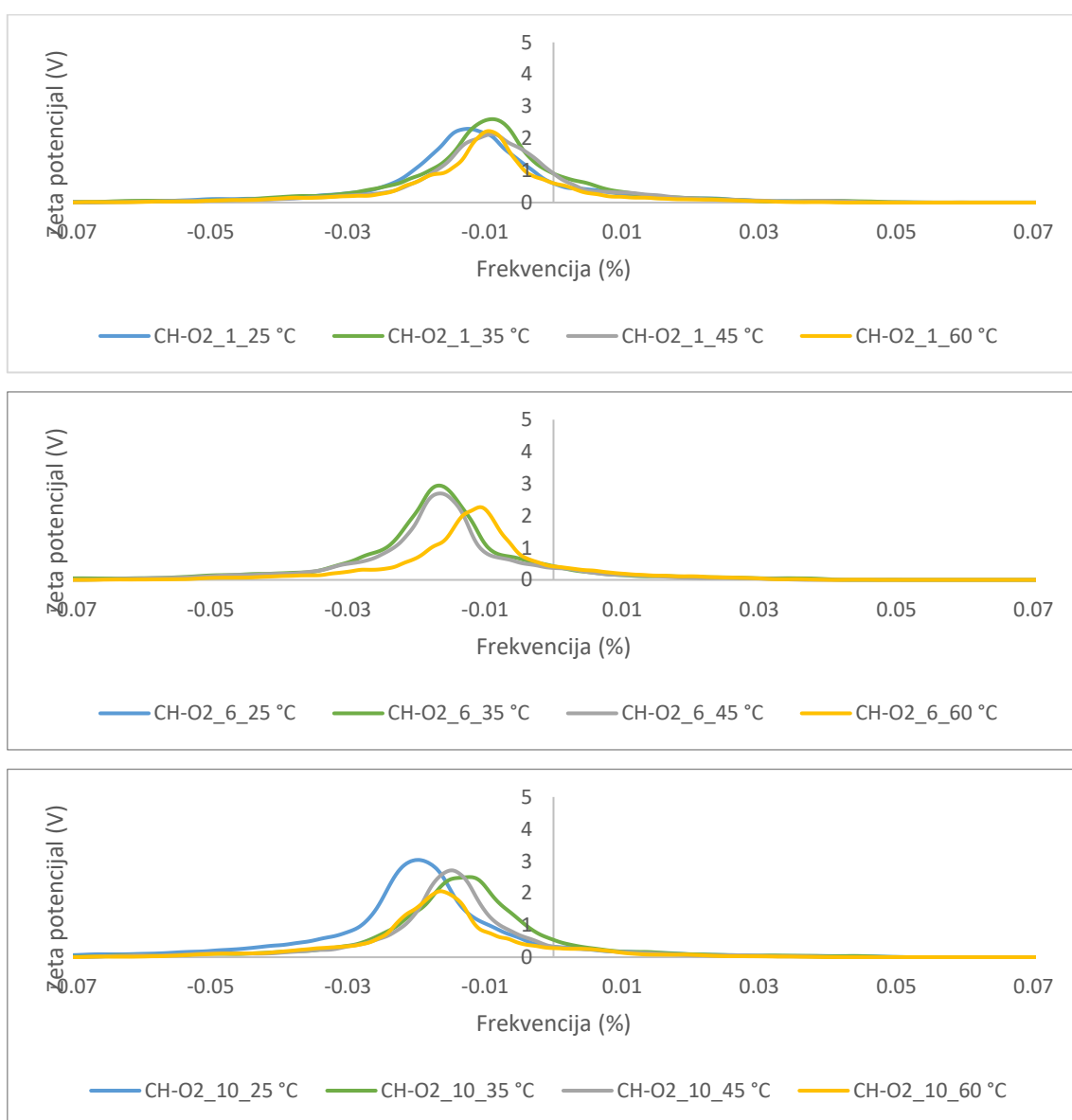
Slika 134. Grafički prikaz krivulje distribucije zeta potencijala ( \zeta ) čestica u efluentu od 1 – 5, 6 – 10 i 1 – 10 ciklusa pranja uzorka CH-P_O 2 pri različitim temperaturama
