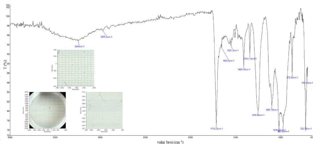
Slika 111. FTIR spekter i mikroskopske slike filtra nakon filtracije efluenta (10 ciklusa pranja) kitozanom modificirane standardne polieterske tkanine predobrađene alkalnom hidrolizom uz dodatak kationskog tenzida
