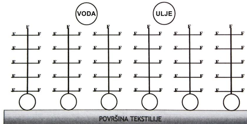
Slika 15. Orijehtacija perfluorovih lanaca na površini tekstilnog materijala
