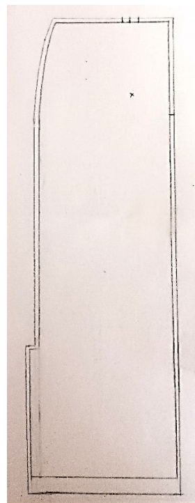
Slika 38, prikaz krojnog dijela sa šavnim dodatcima, stražnjeg donjeg dijela, (Autorica: Nikolina Manda Šarić, kroj rađen po literaturi: Ujević D., Rogale D., Hrastinski M.: Tehnike konstruiranja i modeliranja odjeće – III dopunjeno i prošireno izdanje, Sveučilišni udžbenik, Zrinski Čakovec, 2010.)
