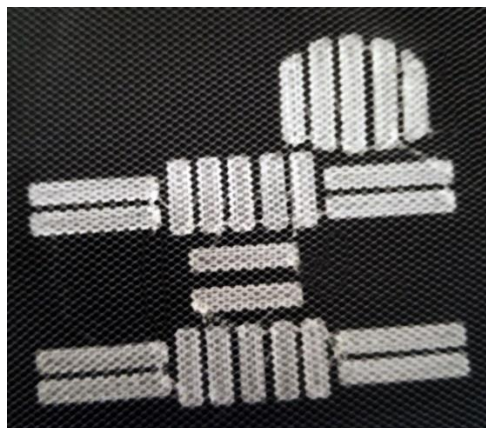
Slika 37. 3D tiskana ojačanja za palac od štapićastih elemenata
