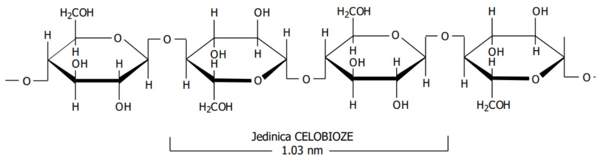
Slika 7: Kemijska formula celuloznog lanca [18]
