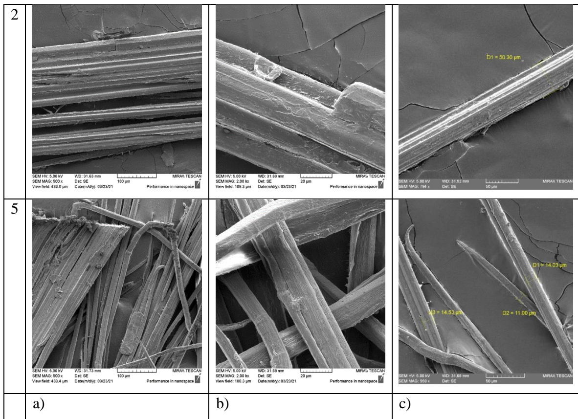
Slika 21. Izgled vlakna nakon obrade 2 s 15% H 2 O 2 te obrade 5 naknadno s 5% NaOH gdje je a) prikaz vlakna pri povećanju 500 x; b) uvećani detalj vlakana pri povećanju 1500 x i c) uvećani detalj vlakana pri povećanju 1500 x na kojem se vidi približna debljina vlakna iz celulozne pulpe.
