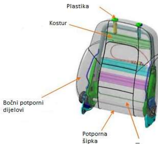
Slika 7. Konstruktivni izgled naslona za leđa [5]
