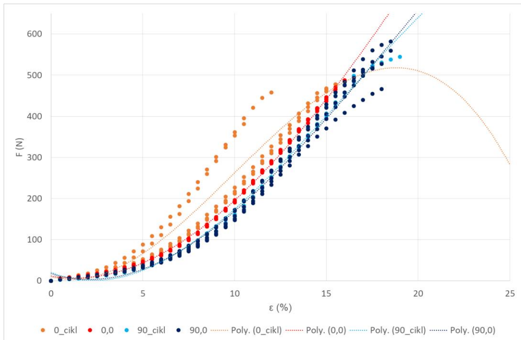
SI. 28. Vlačno ponašanje tkanine u platno vezu (24/24) prije i nakon cikličkog napreznja
