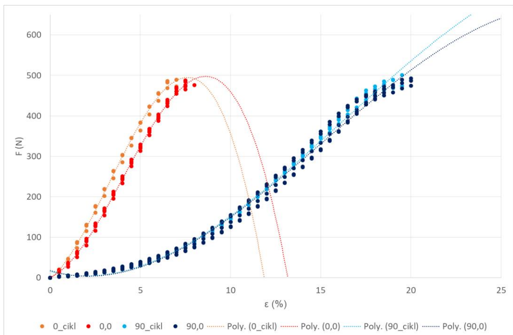
SI. 31. Vlačno ponašanje tkanine u uzdužnom rips vezu (24/24) prije i nakon cikličkog naprezanja
