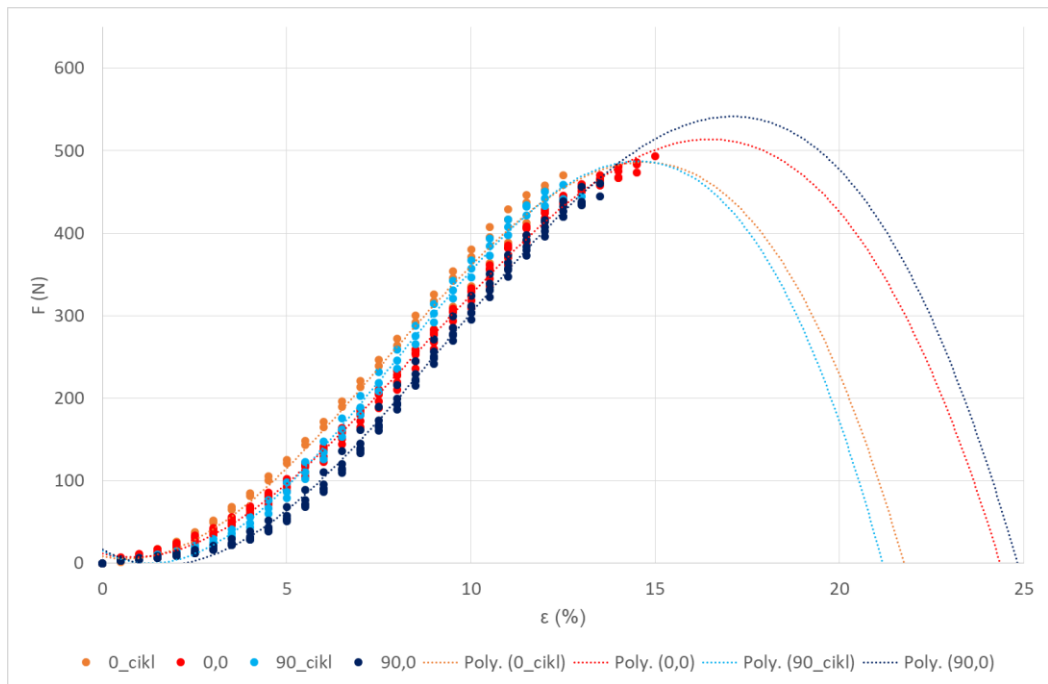
SI. 30. Vlačno ponašanje tkanine u poprečnom rips vezu (24/24) prije i nakon cikličkog naprezanja
