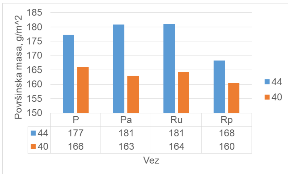
SI. 23. Površinska masa uzoraka tkanina
