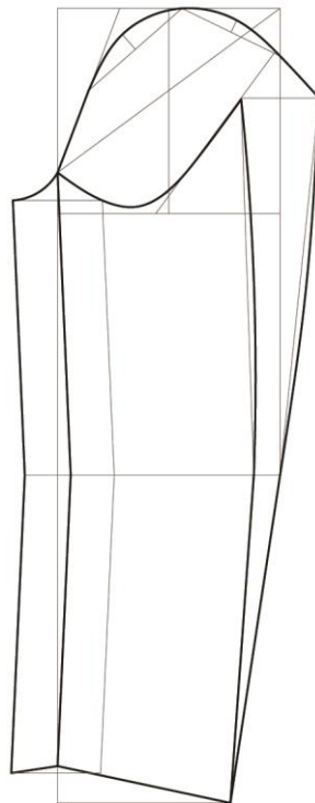
Sl.25.: Konstrukcija rukava za temeljni kroj ženske jakne
