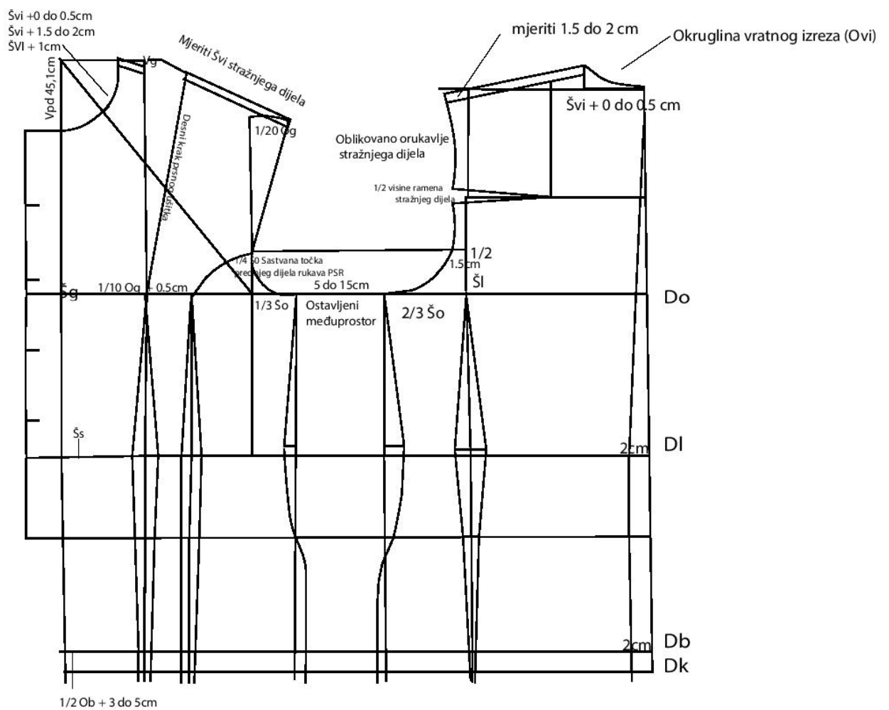
Slika 26. Konstrukcija prednjeg i stražnjeg dijela temeljnog kroja za žensku jaknu
