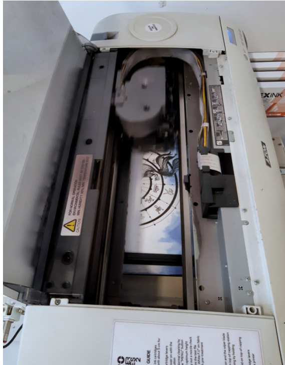
Slika 42: Proces tiskanja na Inkjet Azon TexPro Series2 printeru
