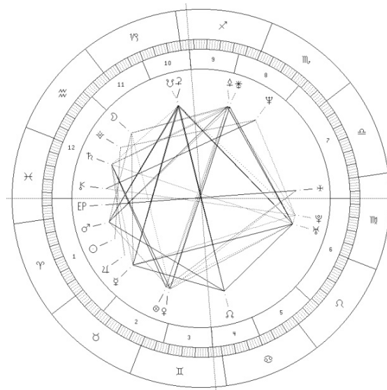
Slika 16: Natalna karta [16]
