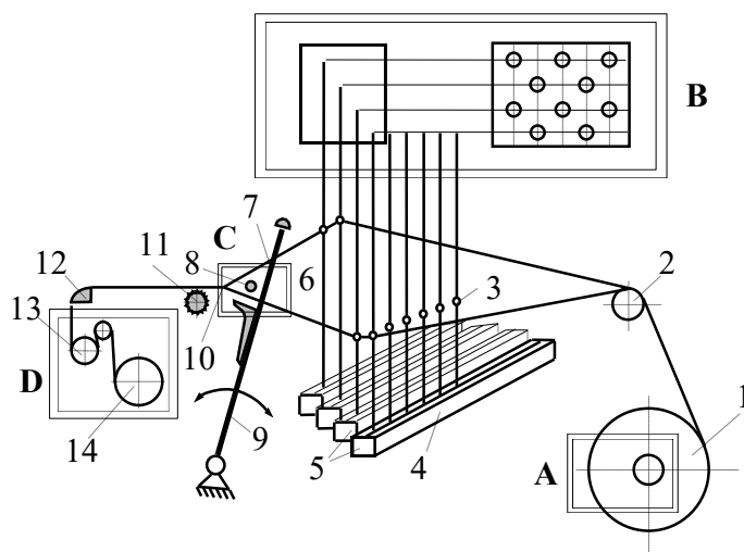
Slika 10. Dijelovi tkalačkog stroja; 1 – osnovin valjak, 2 – prijevojnici, 3 – kotlaci, 4 – listovi, 5 – ničanice, 6 – zijev, 7 – brdo, 8 – potka, 9 – bilo, 10 – prikajna linija, 11 – raširivač, 12 – prsnica, 13 – povlačni valjak, 14 – robni valjak
