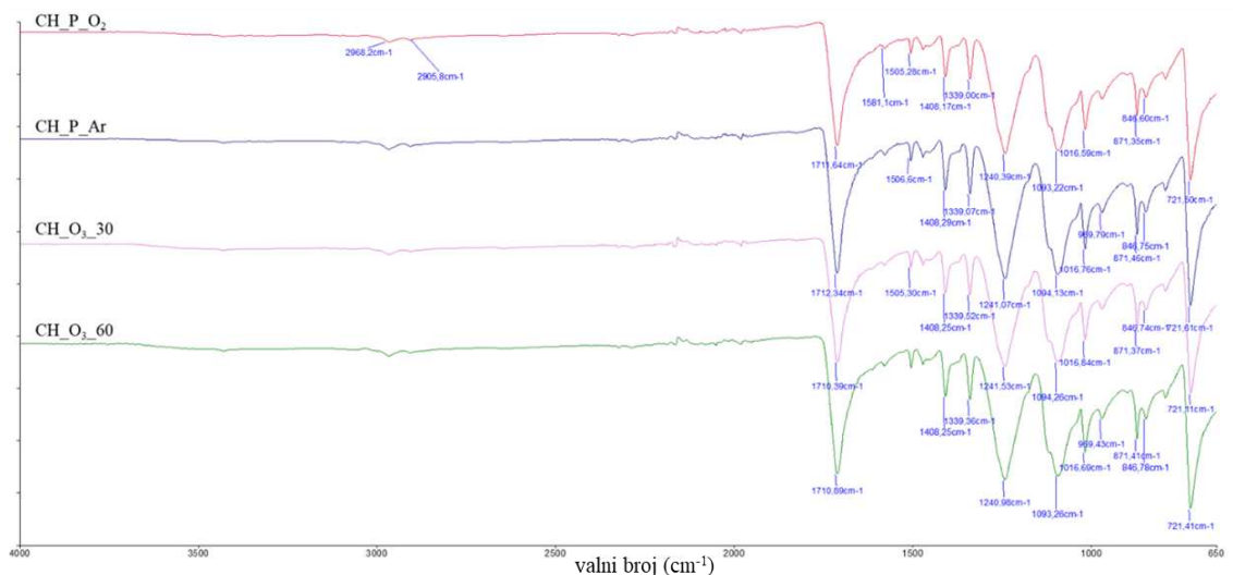
Slika 58. FTIR spektar napredno predobrađene poliesterske tkanine modificirane kitozanom
