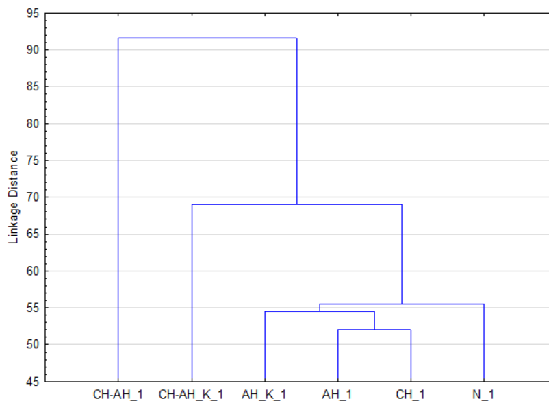
Slika 99. Dendrogram HCA za efluente od 1 – 5 ciklusa pranja konvencionalno predobrađenih i kitozonom modificiranih poliesterskih tkanina
