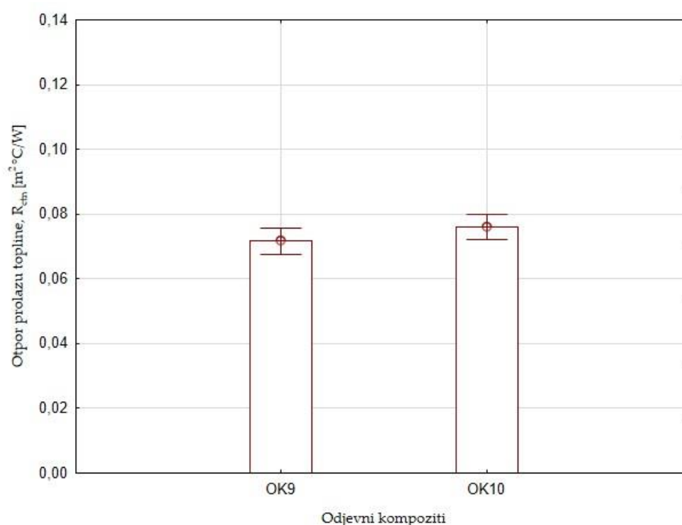
Sl. 60: Raspon srednjih vrijednosti rezultata otpora prolazu topline odjavnog kompozita OK9 (MV2+MP3+MP2) i reprezentativnog odjavnog kompozita OK10 (MV2+MP2+MP3) s naznačenim varijacijama
