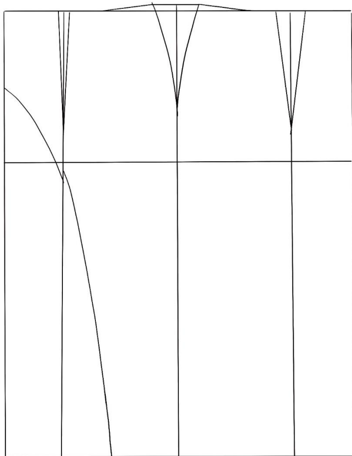
Slika 13. Konstrukcija temeljnog kroja suknje
