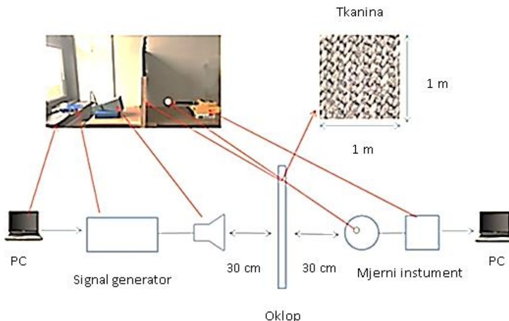
Slika 19. Shematski prikaz mjernog postava [28]
