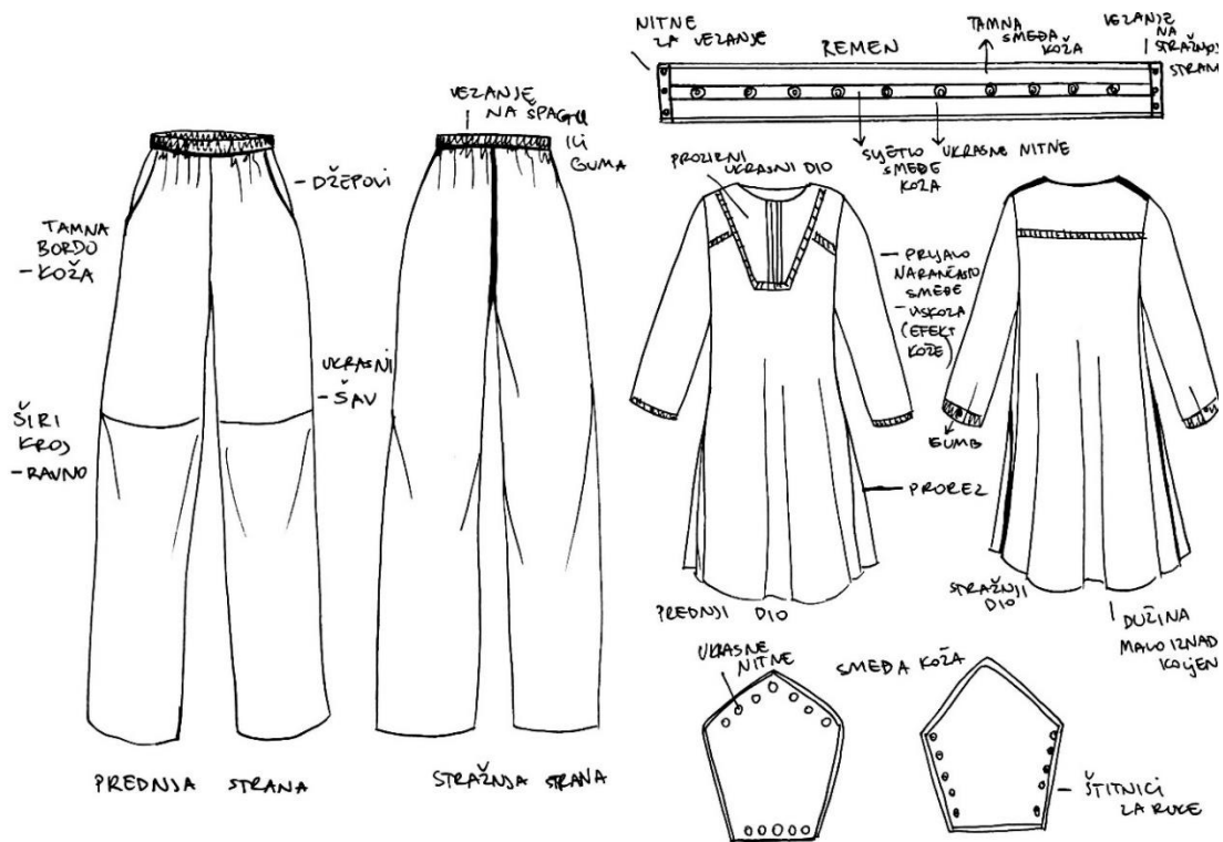
Slika 39. Tehnički crtež za kostim Kriga Ravglans
