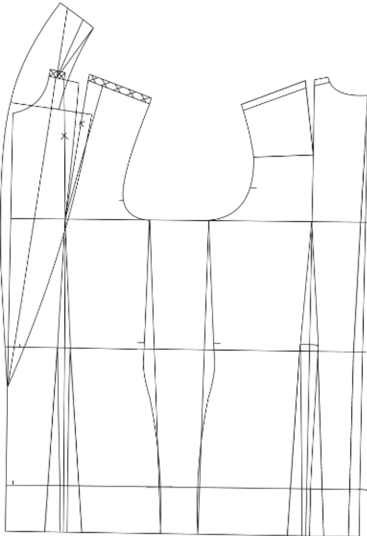
Slika 24 Osnovna konstrukcija sako
