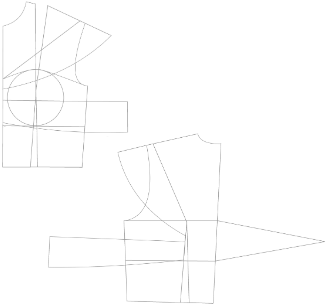
Slika 28 Konstrukcija i modeliranje topa
