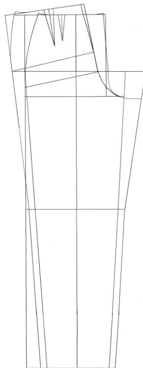
Slika 47: Temeljna konstrukcija ženskih hlača
