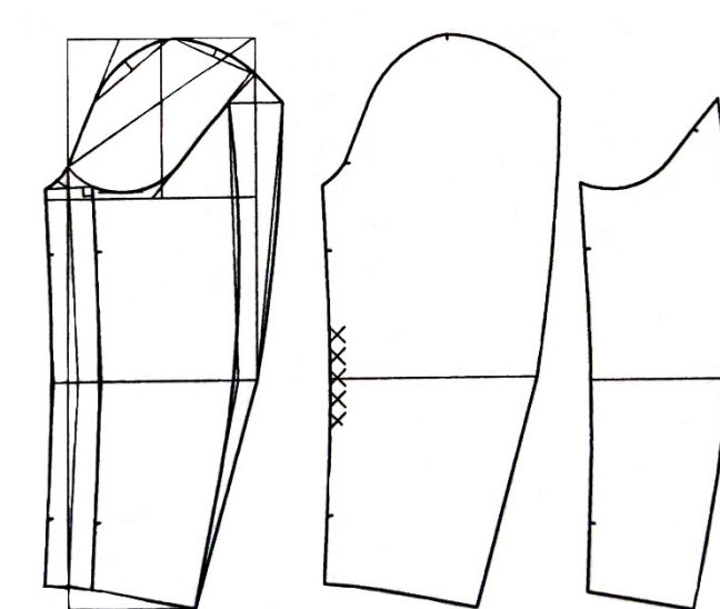
Slika 67. Konstrukcija temeljnog kroja rukava
