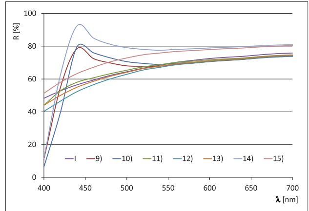
Sl.8 Remisijne krivulje platna opranog tenzidom, tiskanog kombinacijom pasta uz dodatak fluorescentnog optičkog bjelila i fosforescentnog pigmenta
