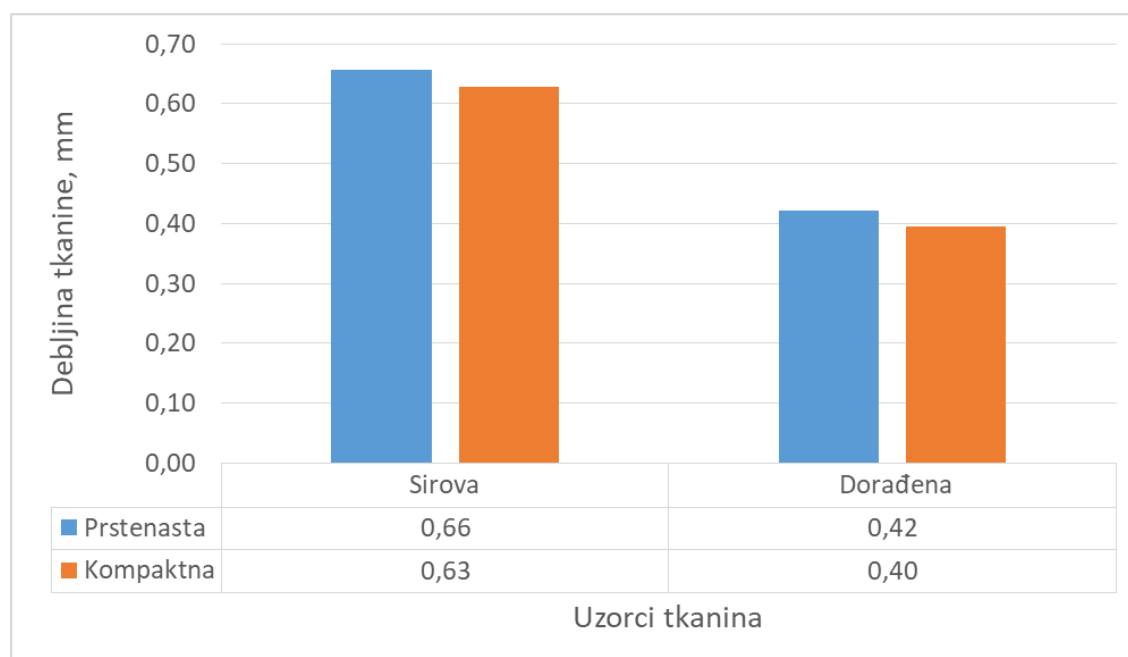
Sl. 30. Debljina tkanina
