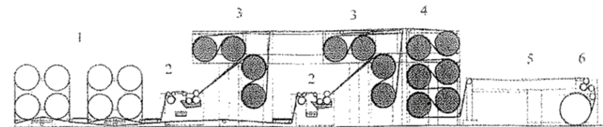
Sl. 9. Shema stroja za škrobljenje s dva korita tt. Sucker Müller Hacoba [16]; 1 – stalak za snovaće valjke, 2 – korito za škrobljenje, 3 – sušionici za sušenje pola osnove, 4 – sušionik za sušenje cijele osnove, 5 – suha podjela osnove, 6 – namatanje škrobljene osnove na osnovin valjak
