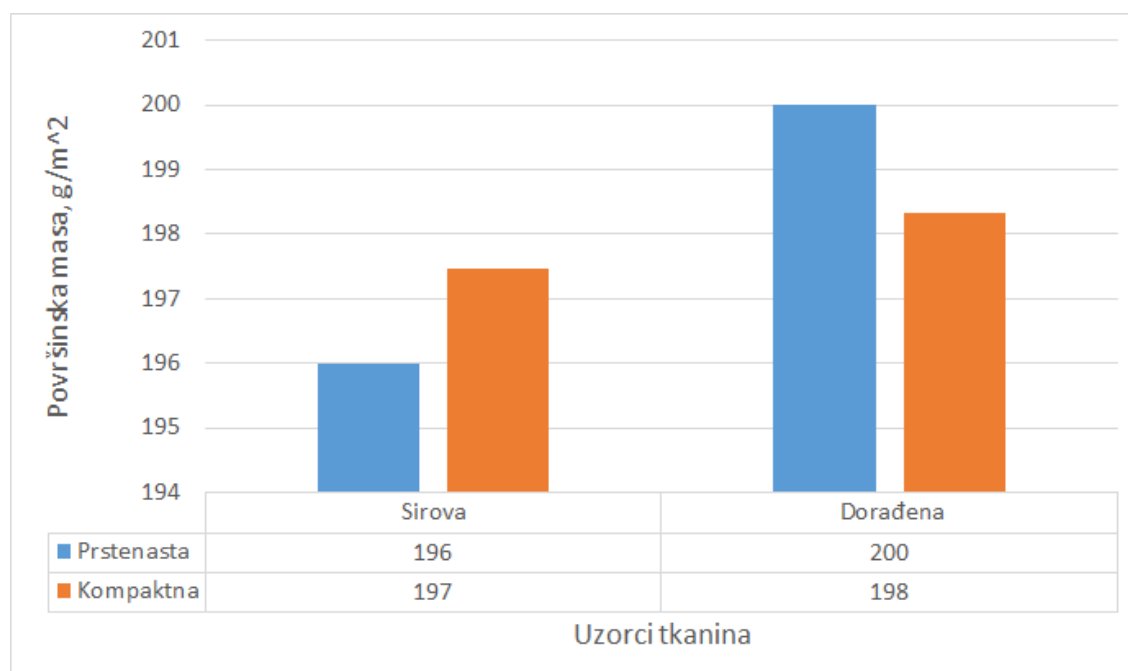
Sl. 31. Površinska masa uzoraka tkanina
