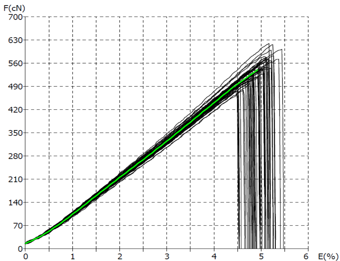
Sl. 26. Vlačne karakteristike prstenaste pređe
