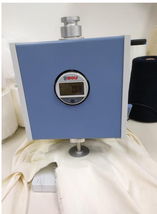
Sl. 25. Debljinomjer
