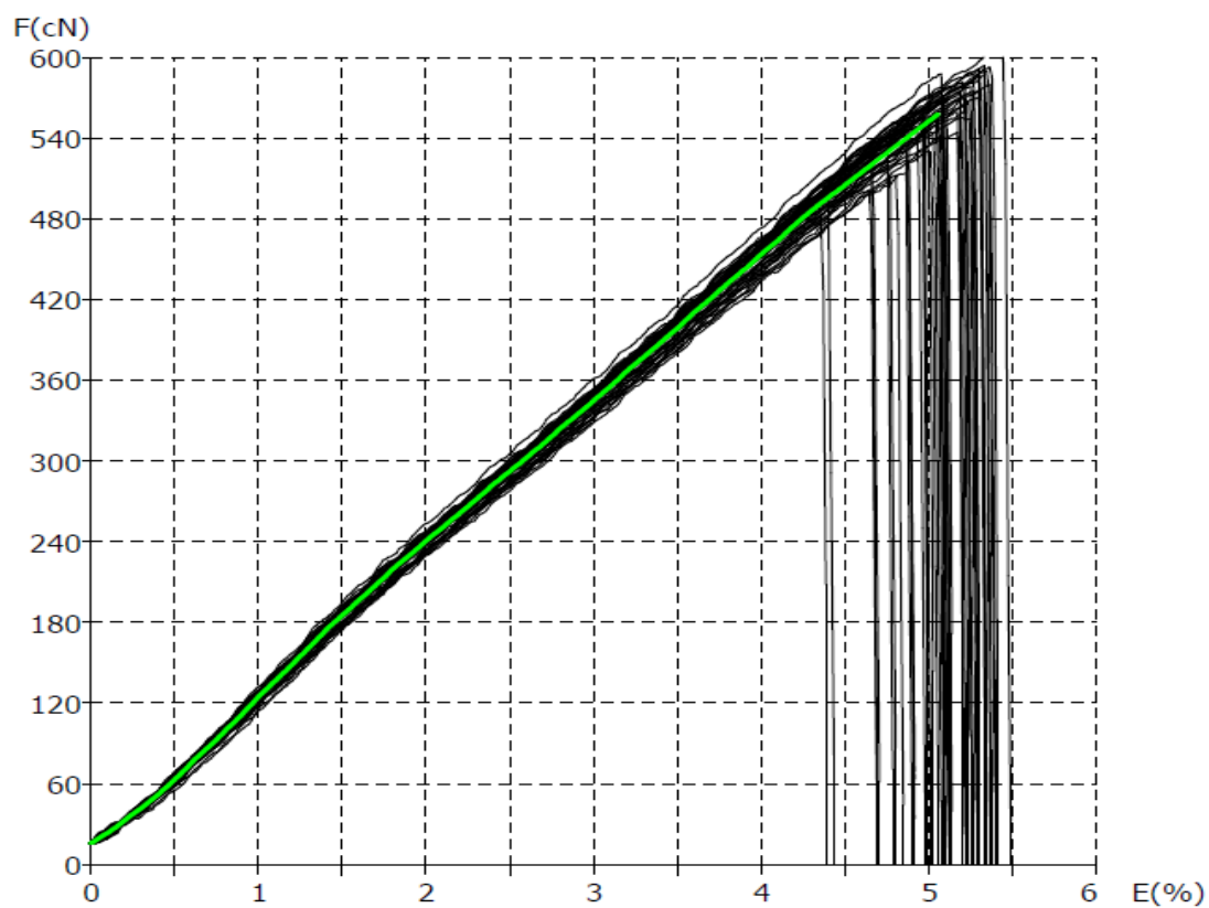
Sl. 27. Vlačne karakteristike kompaktne pređe
