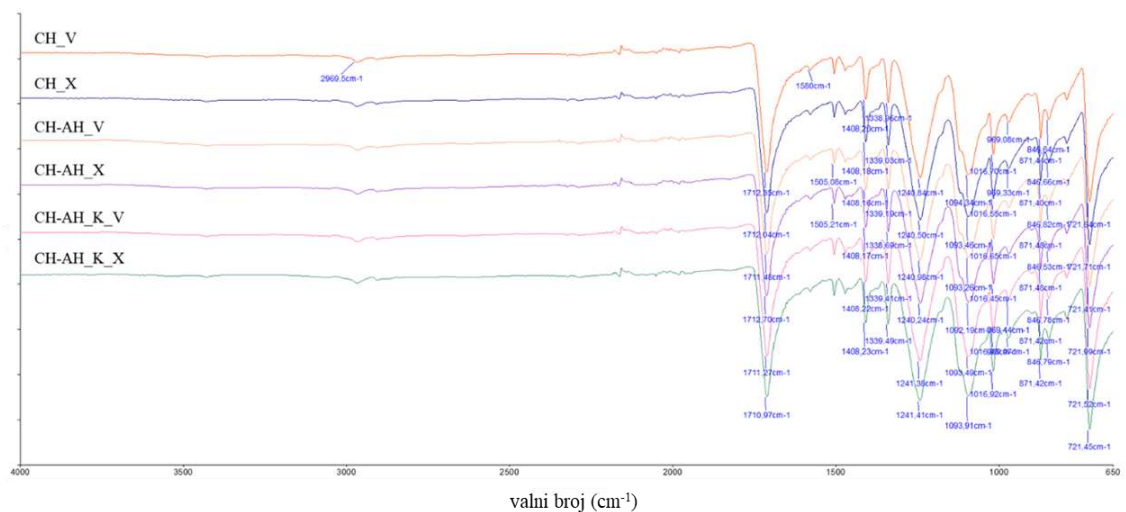
Slika 69. FTIR spektar konvencionalno predobrađene poliesterske tkanine modificirane kitozanom nakon 5 i 10 ciklusa pranja
