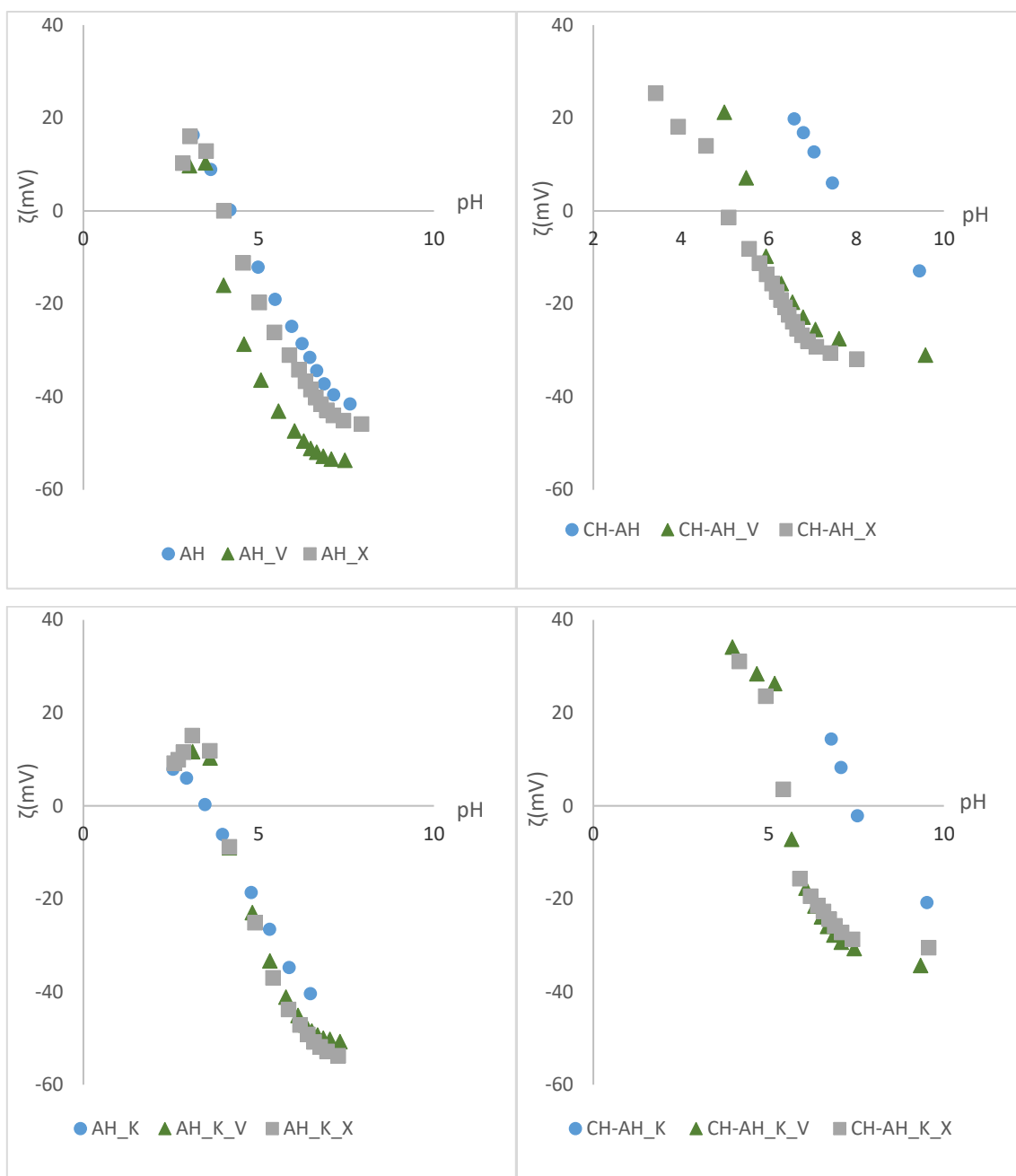
Slika 65. Krivulja zeta potencijala poliesterske tkanine predobrađene konvencionalnim postupcima prije i nakon modifikacije kitozonom nakon 5 i 10 ciklusa pranja u ovisnosti o pH 1 mmol/L KCl
