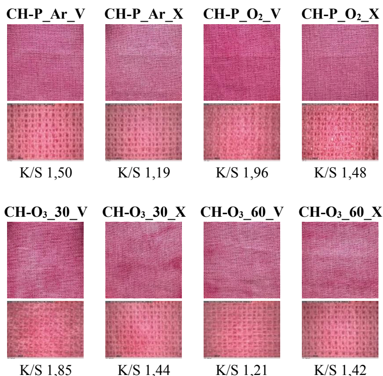
Slika 68. Fotografije snimljene fotoaparatom i Dino lite mikroskopom uz povećanje 50x te K/S vrijednosti napredno predobrađene poliesterske tkanine modificirane kitozanom nakon 5 i 10 ciklusa pranja, nakon identifikacije kitozana bojadisanjem
