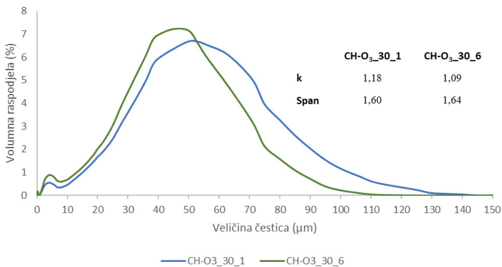
Slika 94. Raspodjela veličina čestica u efluentima od 1 – 5 i 6 – 10 ciklusa pranja polimer/kitozan strukture pripravljene predobradom ozonom u trajanju 30 minuta
