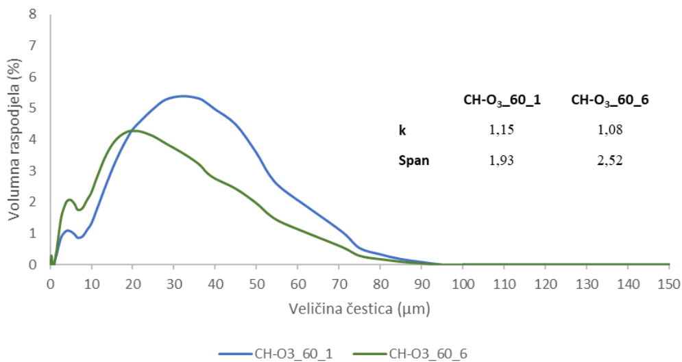
Slika 95. Raspodjela veličina čestica u efluentima od 1 – 5 i 6 – 10 ciklusa pranja polimer/kitozan strukture pripravljene predobradom ozonom u trajanju 60 minuta
