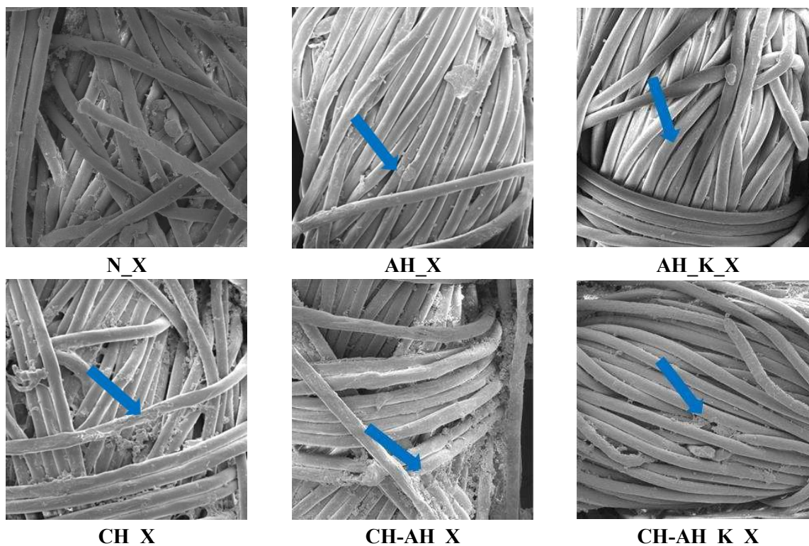
Slika 74. SEM slike nakon 10 ciklusa pranja polieterske tkanine i konvencionalno predobrađene polieterske tkanine prije i nakon modifikacije kitozanom
