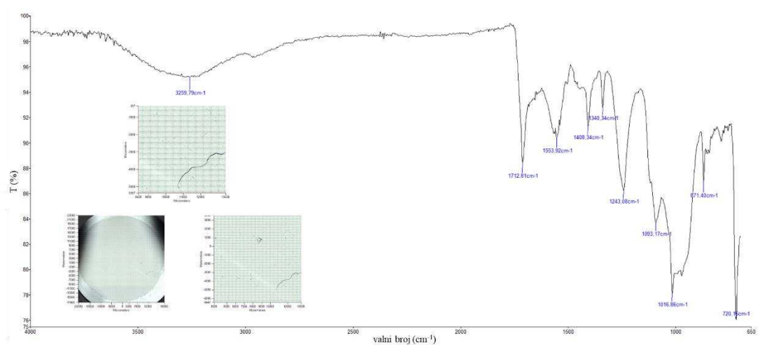
Slika 107. FTIR spektar i mikroskopske slike filtra nakon filtracije efluenta (10 ciklusa pranja) kitozanom modificirane standardne poliesterske tkanine
