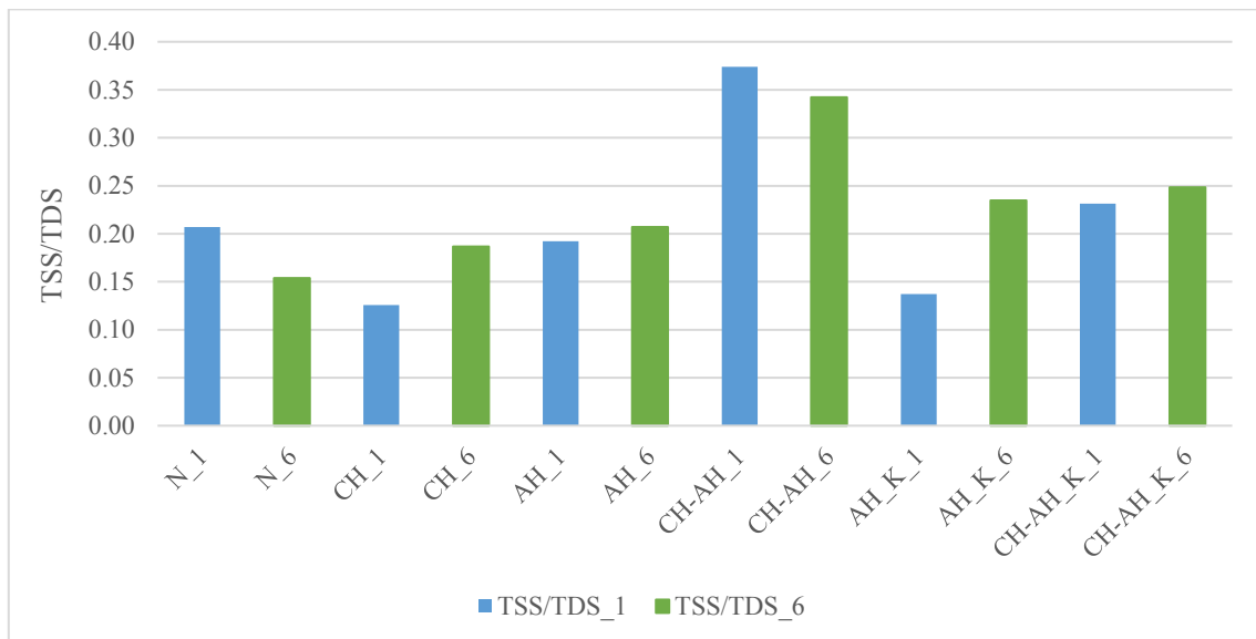
Slika 83. Omjer ukupne suspendirane i ukupne otopljene tvari u efluentima od pranja konvencionalnim predobradama dobivene poliester/kitozan strukture tijekom 1 – 5 i 6 – 10 ciklusa pranja
