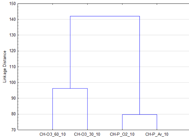
Slika 104. Dendrogram HCA za kompozitne efluente od 10 ciklusa pranja napredno predobrađene poliesterske tkanine modificirane kitozonom
