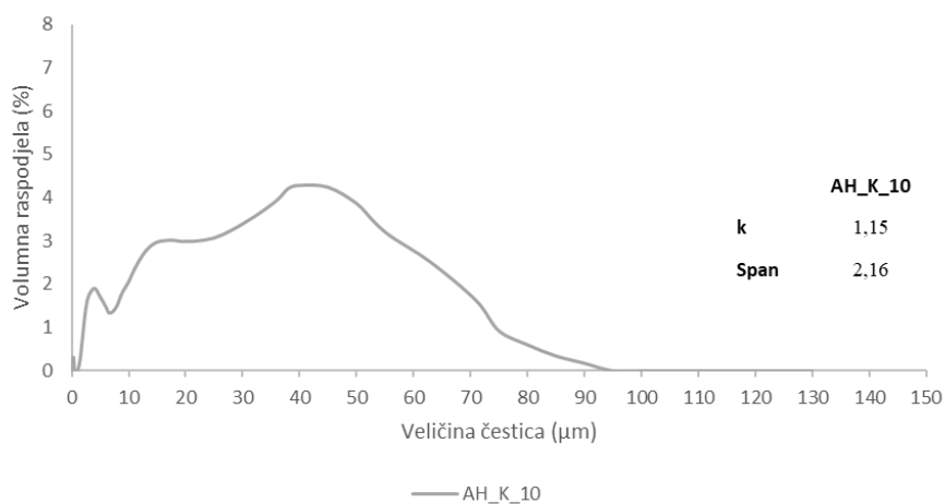
Slika 119. Raspodjela veličina čestica u efluentima od 10 ciklusa pranja alkalno hidrolizirane polieterske tkanine uz dodatak promotora
