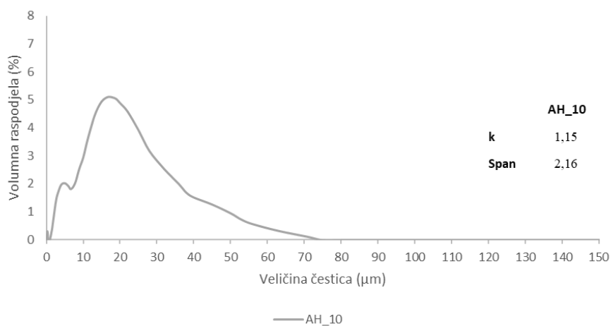
Slika 118. Raspodjela veličina čestica u efluentima za 10 ciklusa pranja alkalno hidrolizirane polieterske tkanine
