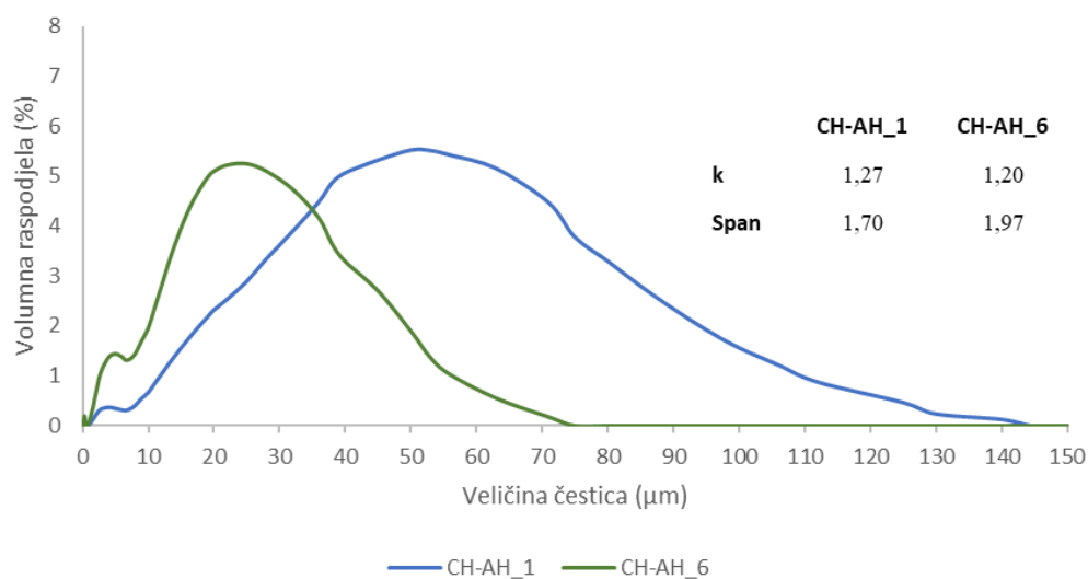
Slika 90. Raspodjela veličina čestica u efluentima od 1 – 5 i 6 – 10 ciklusa pranja poliestester/kitozan strukture pripravljene konvencionalnom predobradom alkalnom hidrolizom
