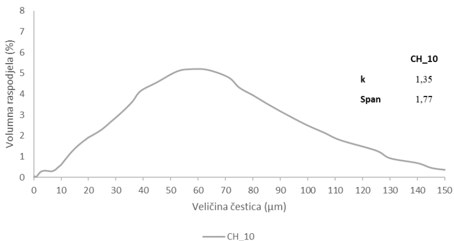
Slika 117. Raspodjela veličina čestica u efluentima za 10 ciklusa pranja kitozonom modificirane polieterske tkanine
