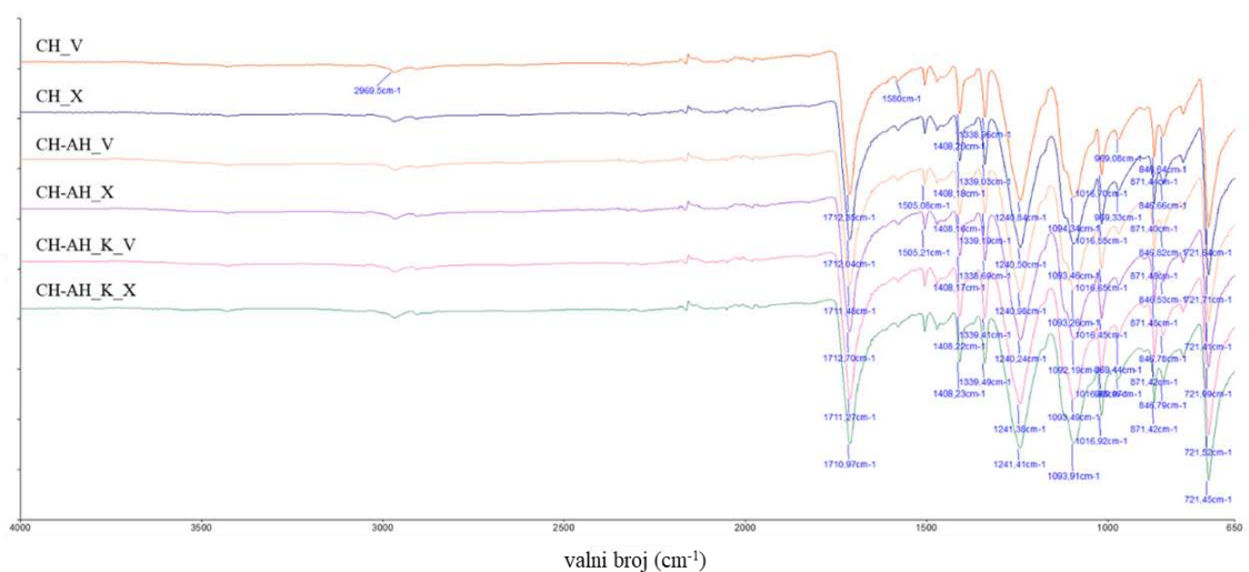
Slika 69. FTIR spektar konvencionalno predobrađene poliesterne tkanine modificirane kitozonom nakon 5 i 10 ciklusa pranja
