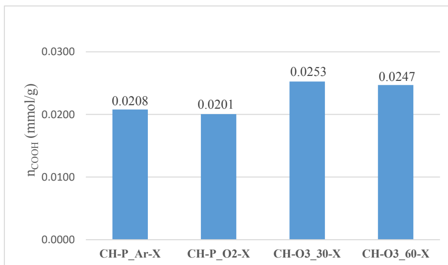
Slika 73. Rezultati analize spektrofotometrijskog određivanja sadržaja karboksilnih skupina iskazanog kao n_{\text{COOH}} napredno predobrađenih poliesterskih tkanina modificiranih kitozonom
