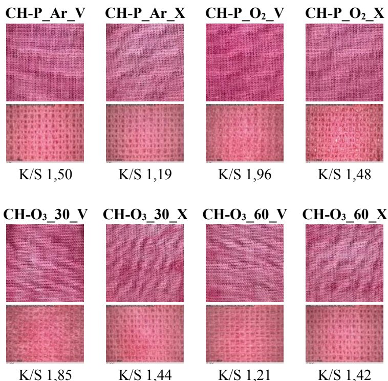
Slika 68. Fotografije snimljene fotoaparatom i Dino lite mikroskopom uz povećanje 50x te K/S vrijednosti napredno predobrađene poliesterne tkanine modificirane kitozonom nakon 5 i 10 ciklusa pranja, nakon identifikacije kitozana bojadisanjem
