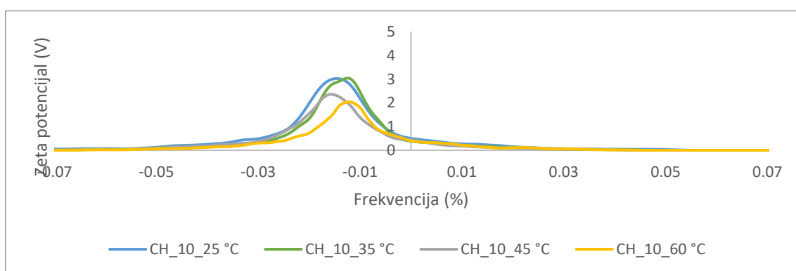
Slika 130. Grafički prikaz krivulje distribucije zeta potencijala ( \zeta ) čestica u efluentu od 1 – 5, 6 – 10 i 1 – 10 ciklusa pranja uzorka CH N pri različitim temperaturama
