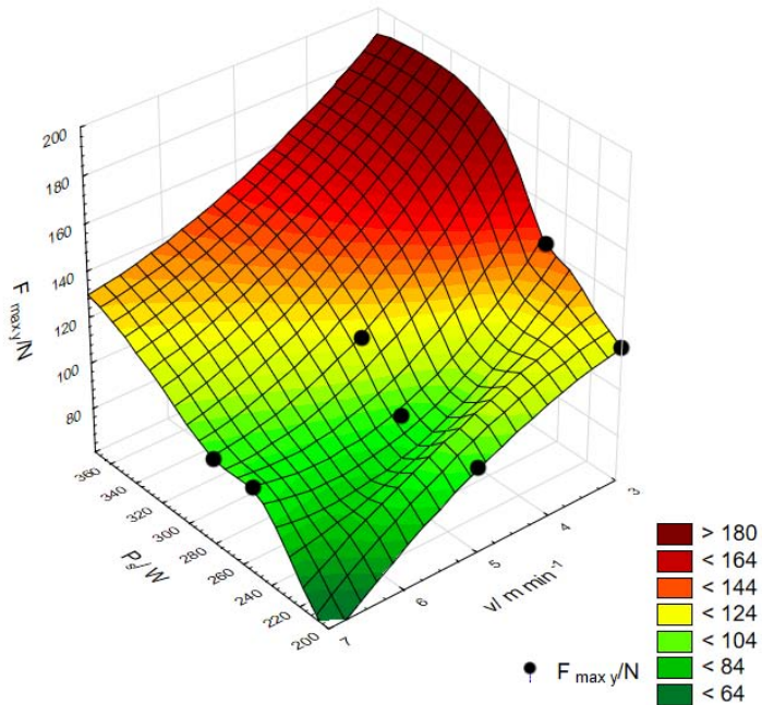
SI. 4.57 Prikaz odnosa ultrazvučnih parametara spajanja, brzine spajanja, v_I \text{ m min}^{-1} i snage ultrazvučnog spajanja, P_s/W na čvrstoću spoja F_{\max}/N , spojenog uzorka materijala oznake M10 LL (lice na lice spajanog materijala) u a) x smjeru i b) y smjeru spajanja
