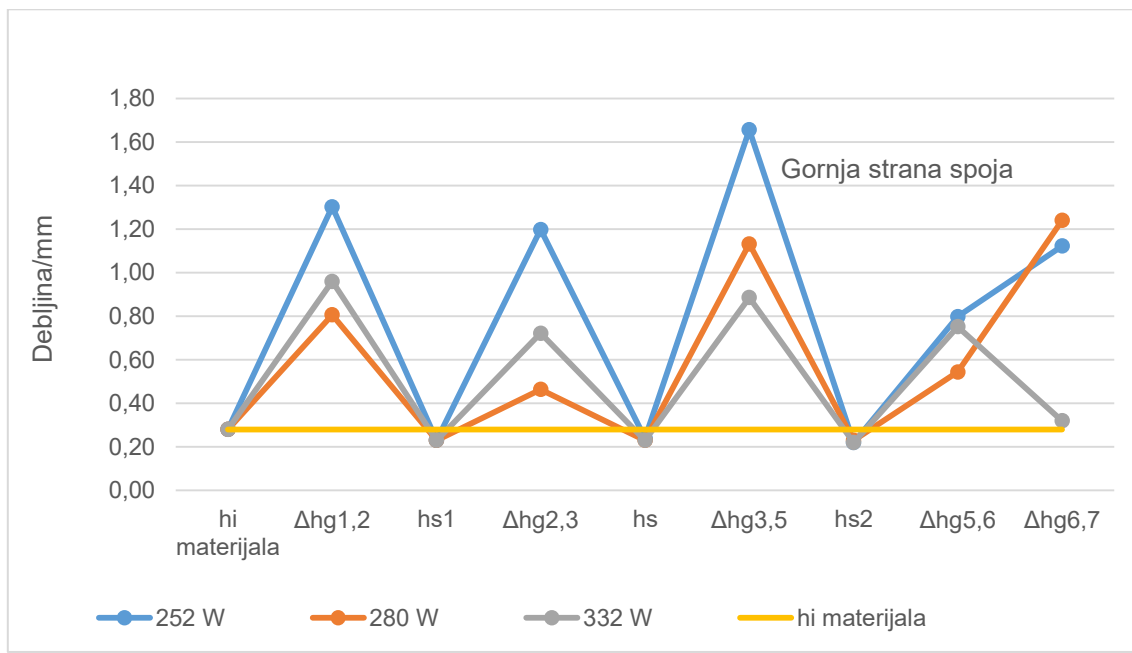
SI. 4.86 Prikaz izmjerenih vrijednosti debljinu izratka, debljina spoja i razlike između vrijednosti debljine spoja i istisnutog ruba za spoj mjereno s gornje strane na uzorku materijala oznake M11, spajano na način NN (naličje na naličje spajano materijala) u y smjeru
