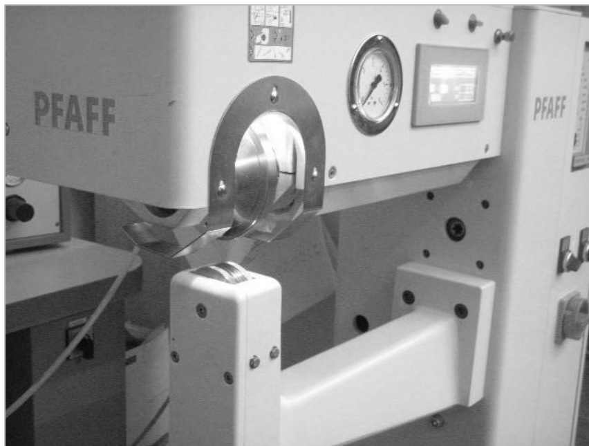
Sl. 3.5 Stroj za ultrazvučno spajanje proizvođača Pfaff oznake Seamsonic 8310-003
