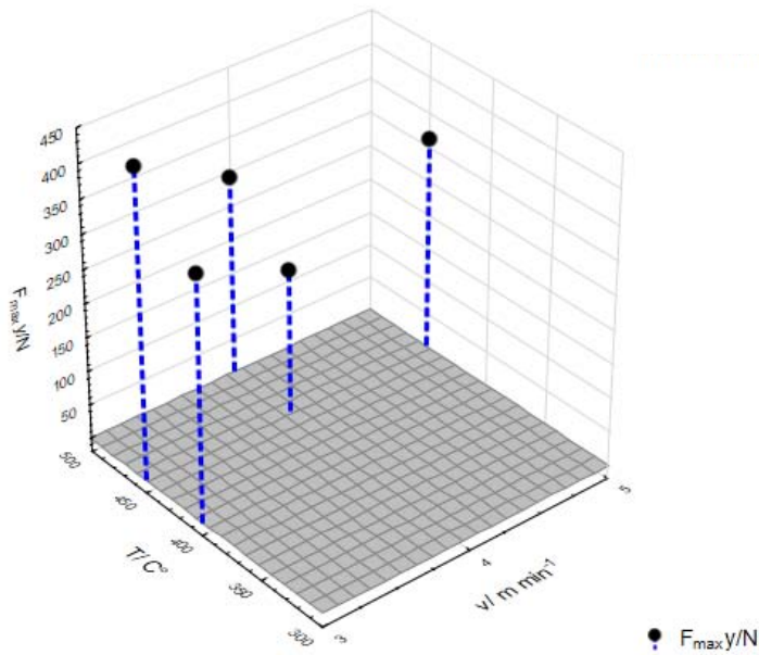
SI. 4.72 Prikaz odnosa parametara spajanja toplinskom kondukcijom, brzina spajanja, v/\text{m min}^{-1} i temperatura vrućeg klina, T/^\circ\text{C} na čvrstoću spoja F_{\text{max}}/\text{N} , spojenog uzorka materijala oznake M10, spajanog na način L1N1 (lice na naličje spajanog materijala) u a) x smjeru; b) y smjeru
