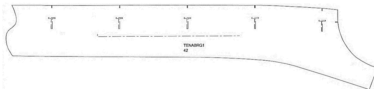
Sl. 151. Krojni dio za bilježenje pozicija rupica za gumbе
