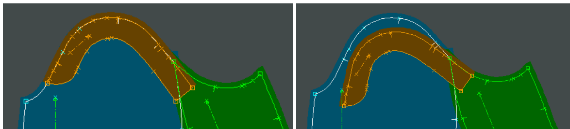
Sl. 131. i 132. Završna kontrola krojnog dijela za vatelin kugle rukava
