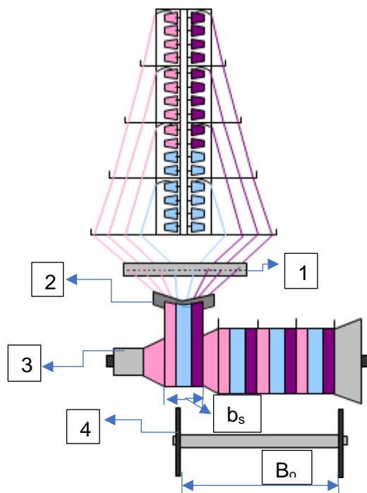
Sl.3. Sekcijsko snovanje: 1 – brdo za prijebore, 2 – snovače krilasto brdo, 3 – sekcijski bubanj, 4 – osnovin valjak, b_s – širina sekcije, B_o – širina osnove na osnovinom valjku [4]
